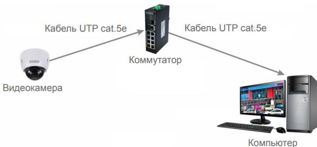
Рисунок 6.3 – Схема подключения видеокamеры к компьютеру через коммутатор
