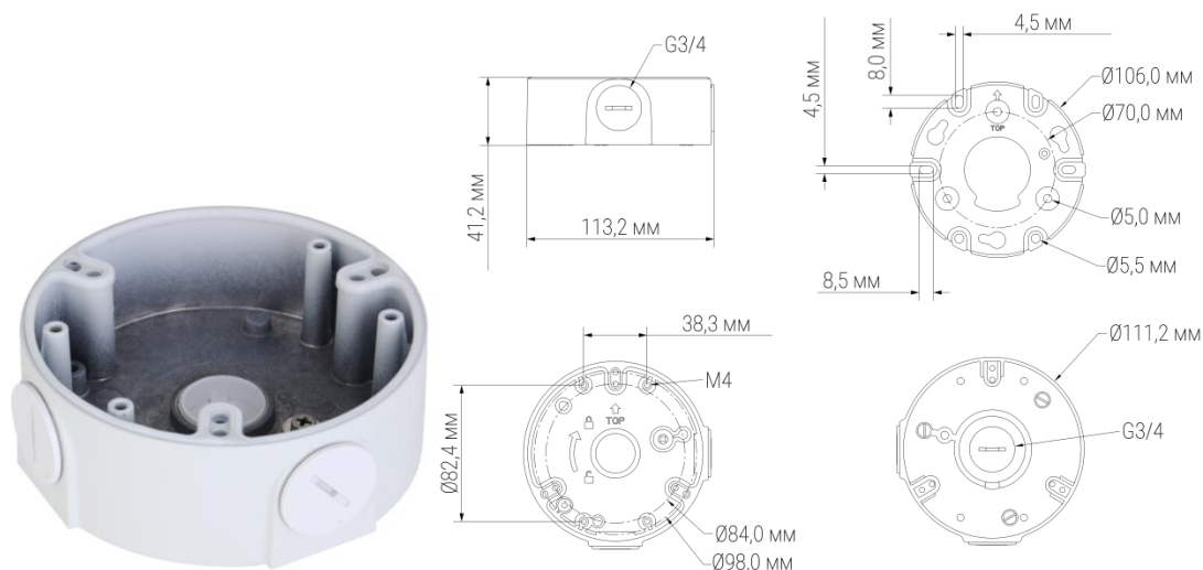
Рисунок 5.6 – Монтажная коробка BR-205
