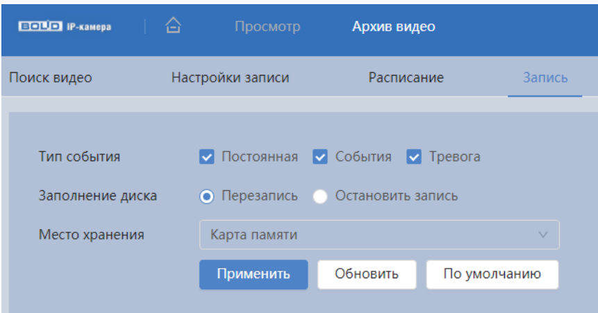
Рисунок 7.90 – Вкладка «Запись»
