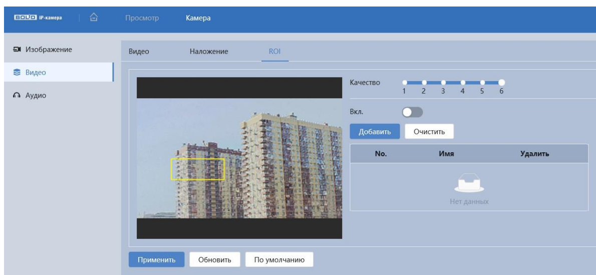
Рисунок 7.46 – Вкладка «ROI»
