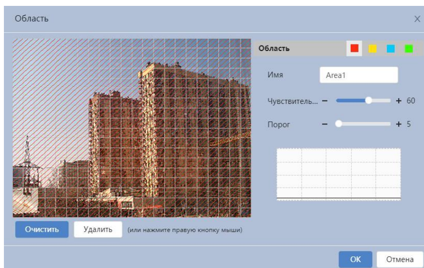
Рисунок 7.59 – Вкладка «Область»
