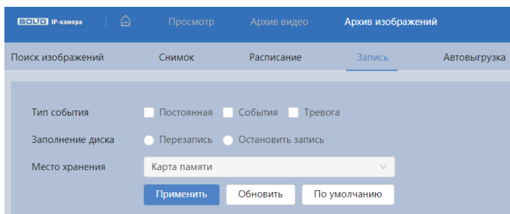
Рисунок 7.96 – Вкладка «Запись»
