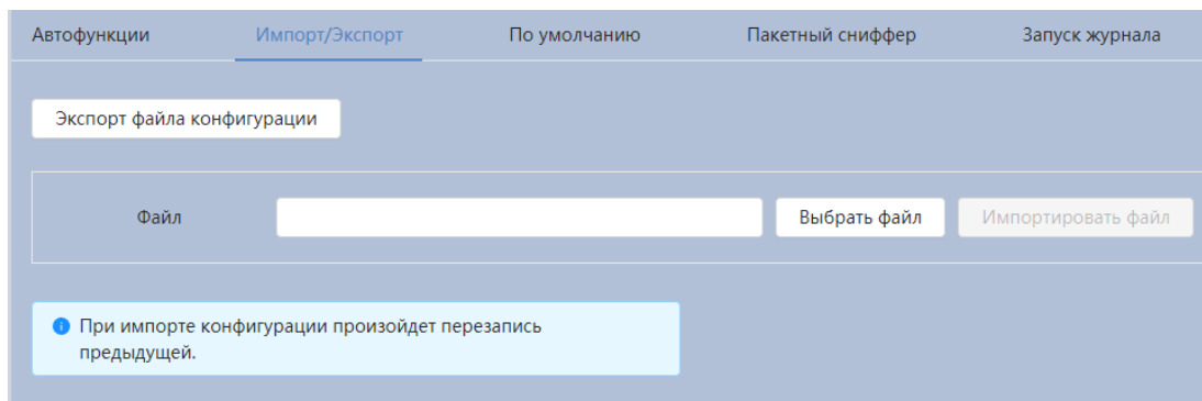
Рисунок 7.78 – Вкладка «Импорт/Экспорт»
