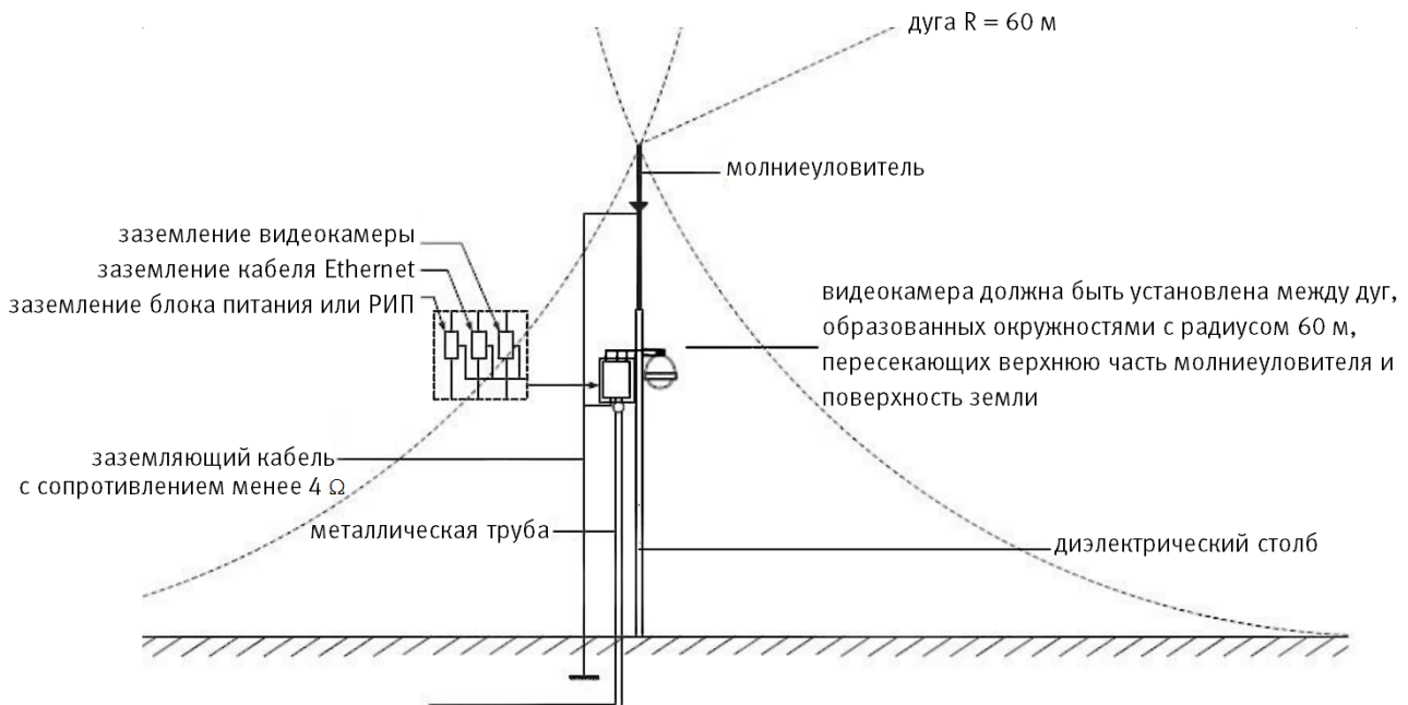
Рисунок 6.13 – Установка молниеотвода
