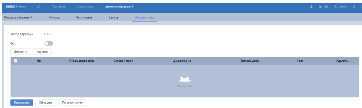
Рисунок 7.99 – Вкладка «Автовыгрузка»
