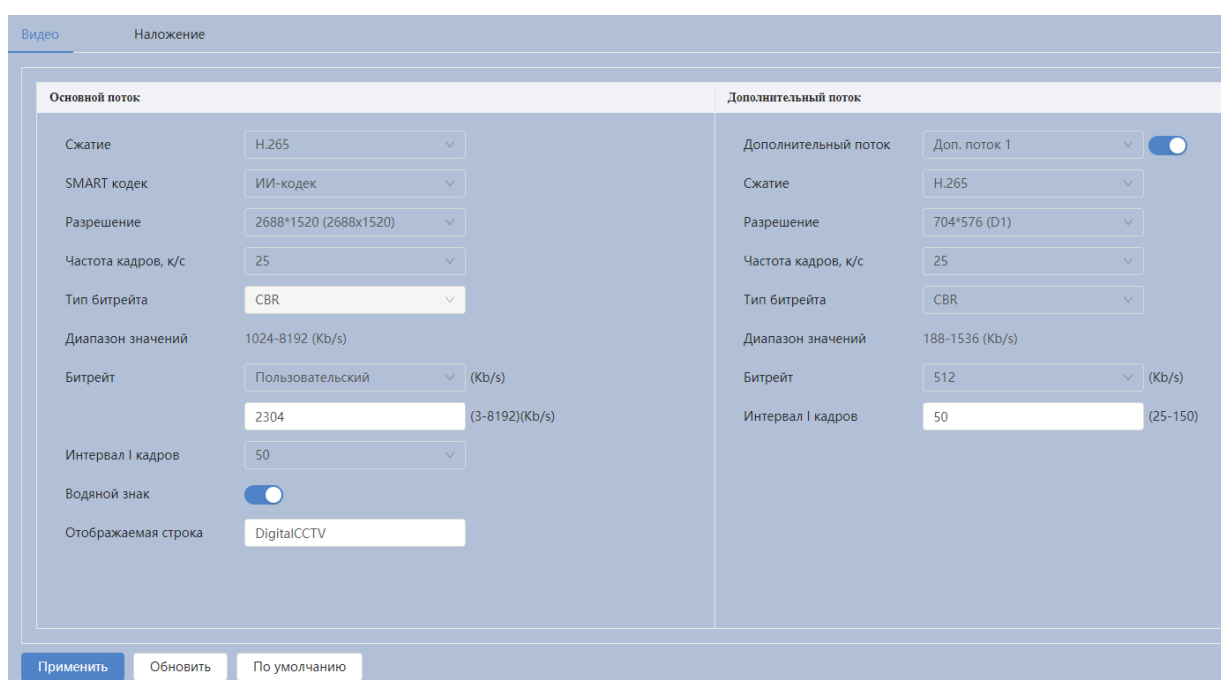
Рисунок 7.38 – Вкладка «Видео»
