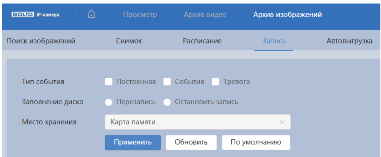
Рисунок 7.97 – Вкладка «Запись»
