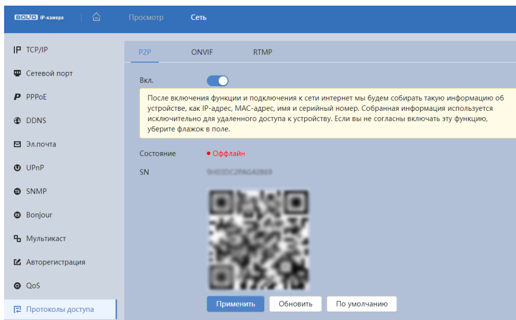
Рисунок 8.19 – Вкладка «P2P»
