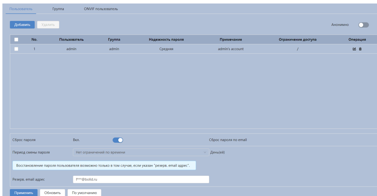
Рисунок 7.72 – Вкладка «Пользователь»
