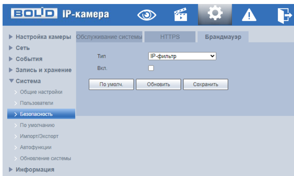
Рисунок 7.121 – Вкладка «Брандмауэр»
