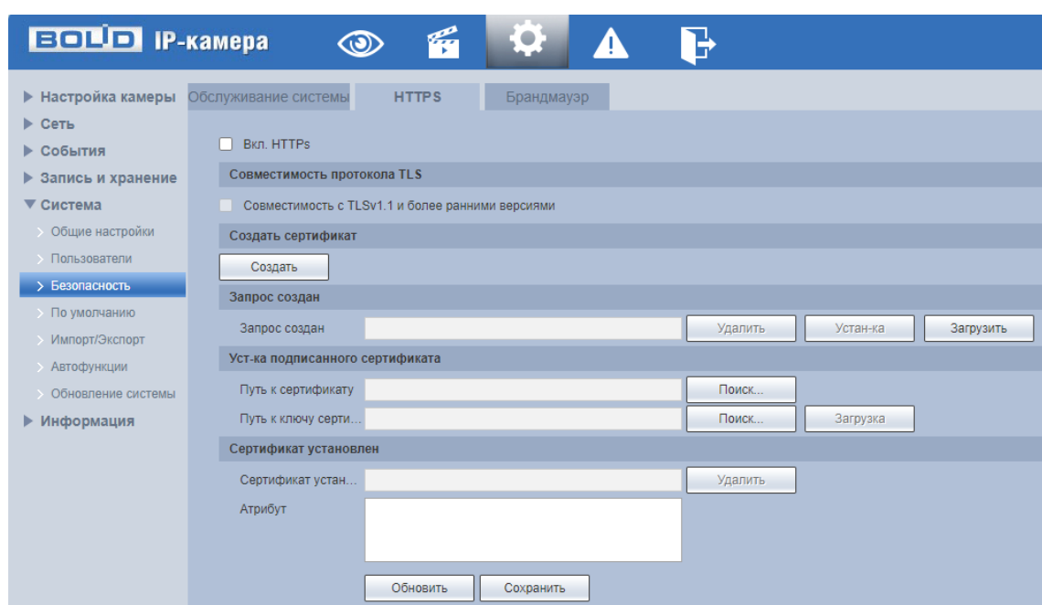
Рисунок 7.119 – Вкладка «HTTPS»
