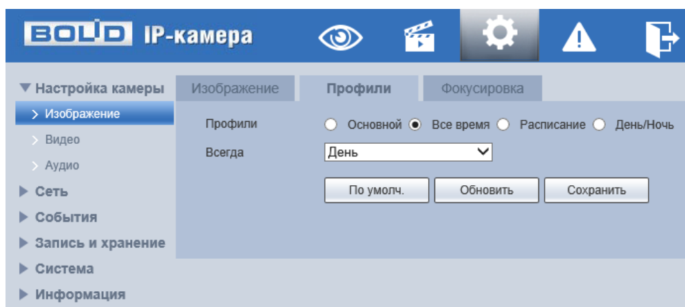
Рисунок 7.36 – Вкладка «Профили»
