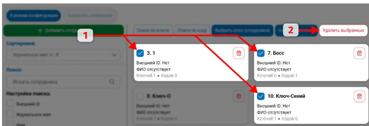
Рисунок 128. Удаление сотрудников
