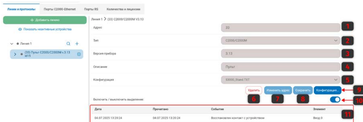
Рисунок 102. Параметры пультов
