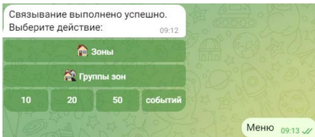
Рисунок 156. Меню бота
