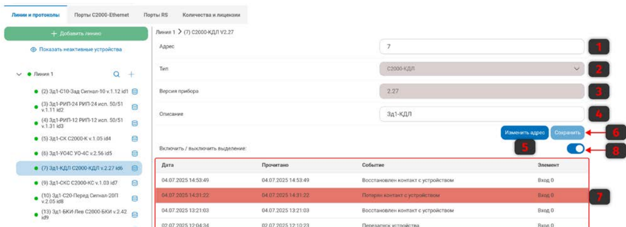
Рисунок 103. Параметры устройств
