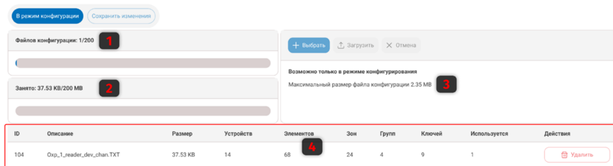
Рисунок 112. Страница «Конфигурации»
