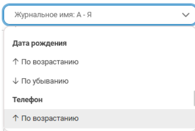
Рисунок 116. Сортировка сотрудников
