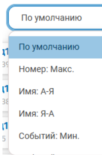
Рисунок 45. Сортировка списка
