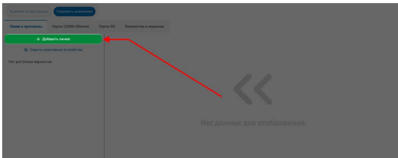
Рисунок 100. Добавление линии
