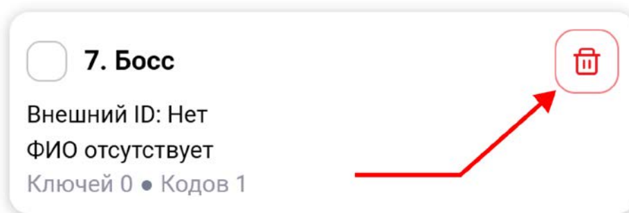
Рисунок 127. Удаление сотрудника
