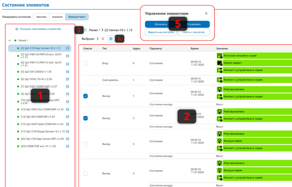
Рисунок 129. Страница «Элементы»
