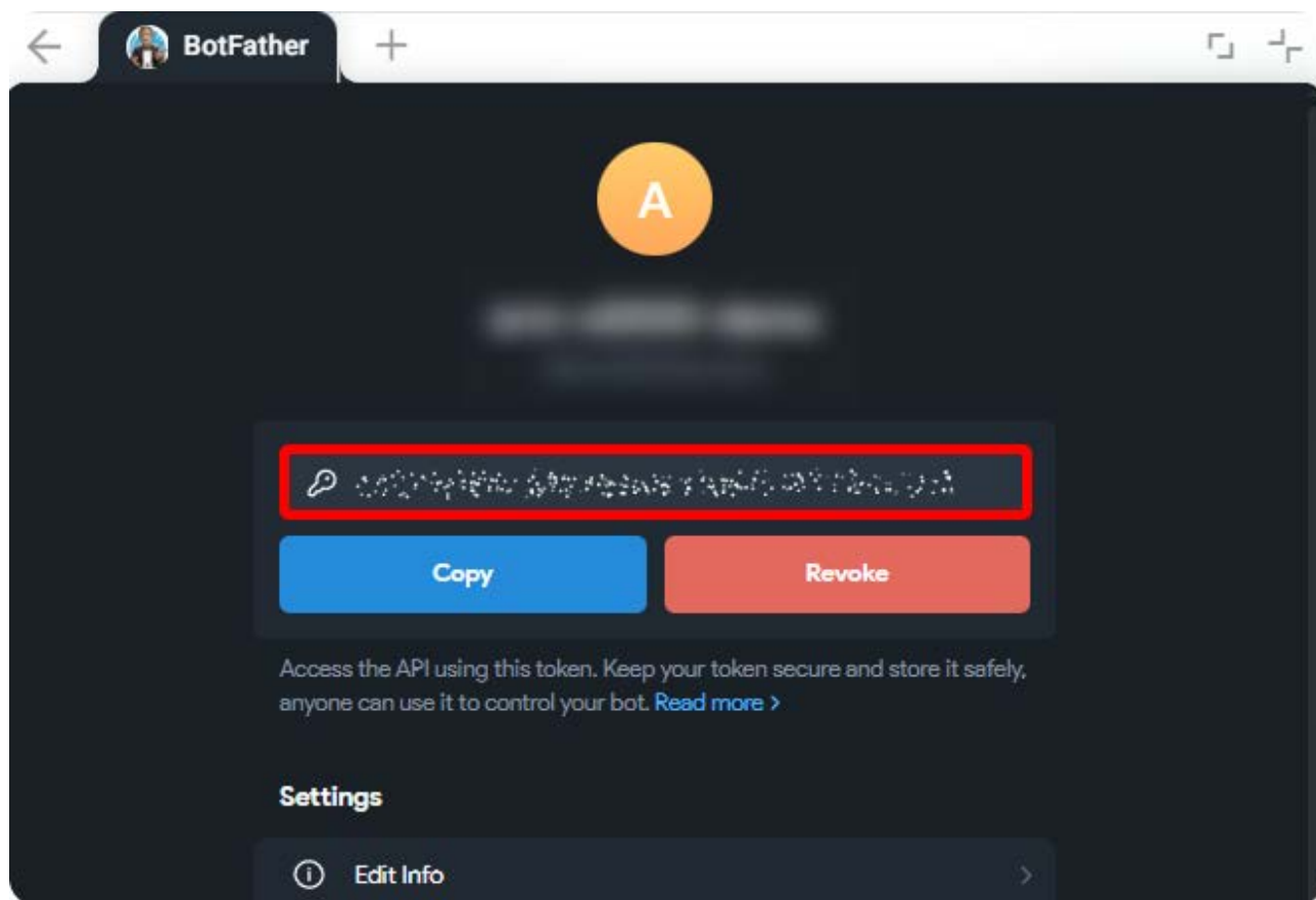
Рисунок 143. Получение токена
