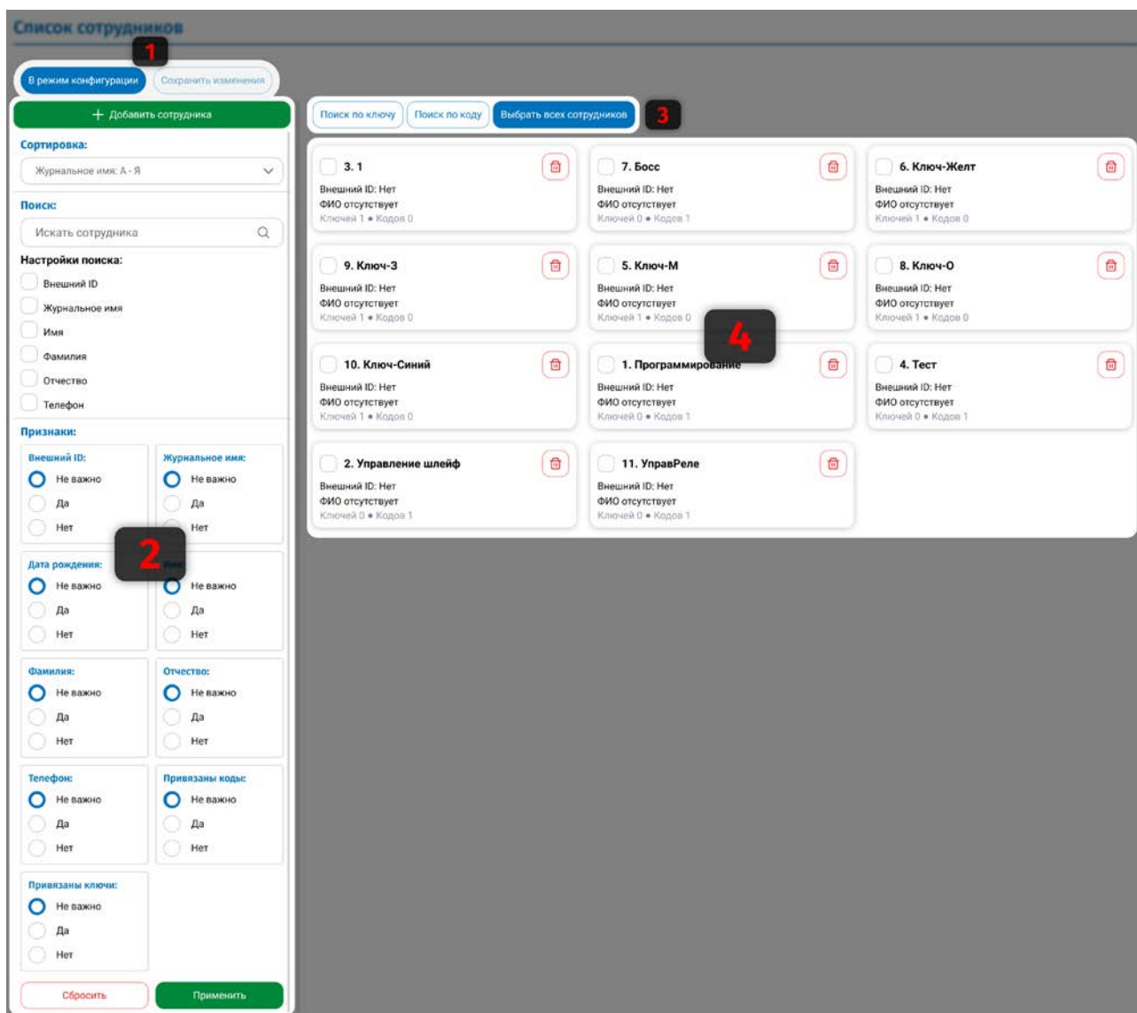
Рисунок 115. Страница «Сотрудники»
