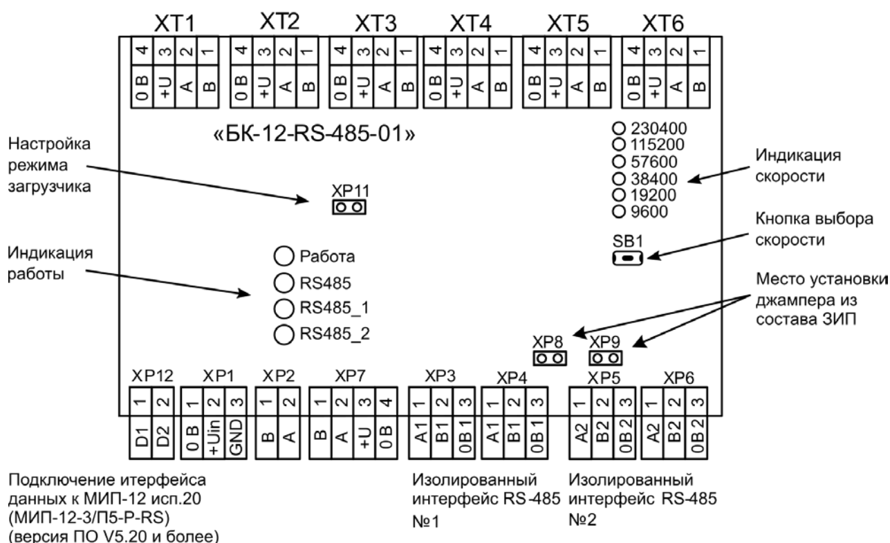
БК-12-RS-485-01 с открытой крышкой
