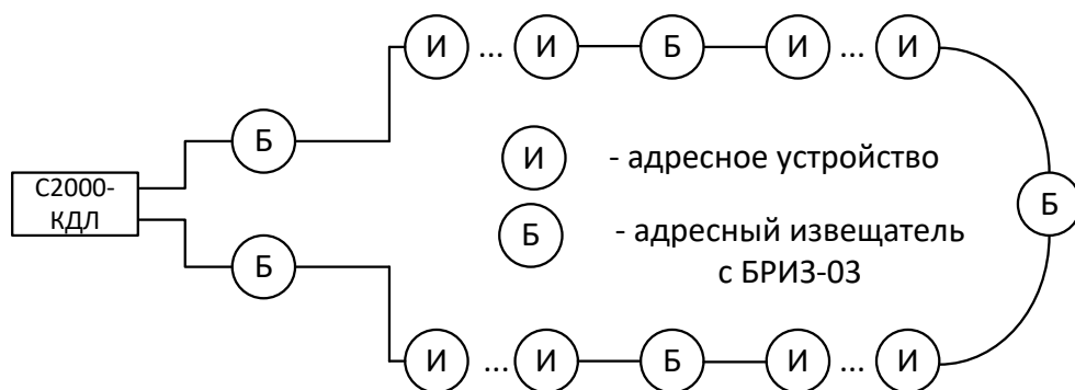
Рисунок 2.2.3 Топология «кольцо»
