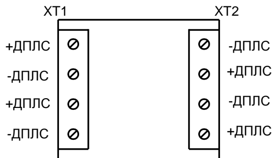
Рисунок 2.2.4.1 Схема подключения.
