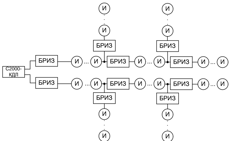
Рисунок 2.2.4 Топология «дерево»
