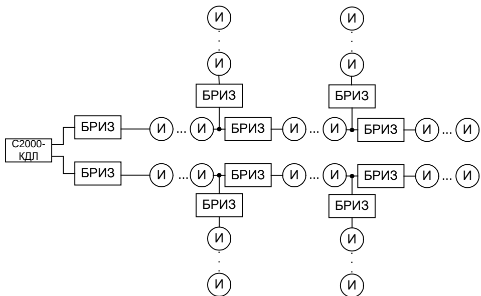
Рисунок 2.2.4 Топология «дерево»
