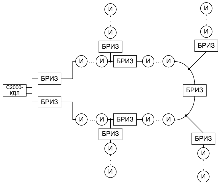
Рисунок 2.2.5 Смешанная топология
