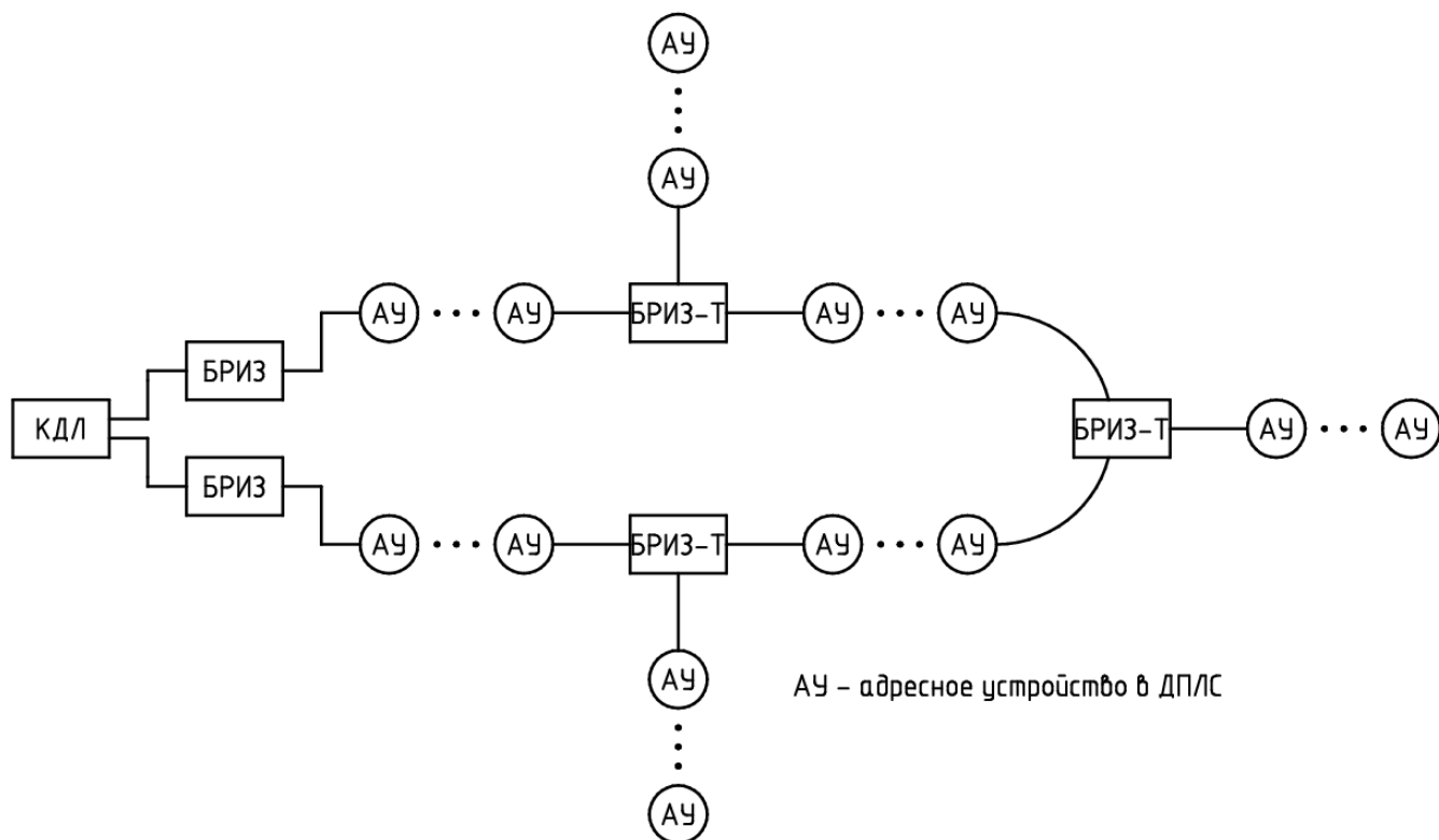
Рисунок 2.2.4.2 Топология смешанного типа
