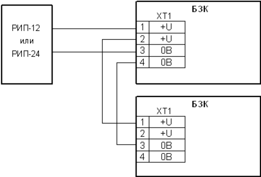
Схема параллельного подключения БЗК
