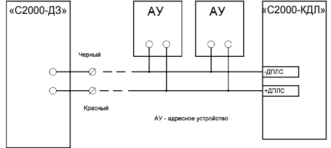
Рисунок 1 – Схема подключения датчика
