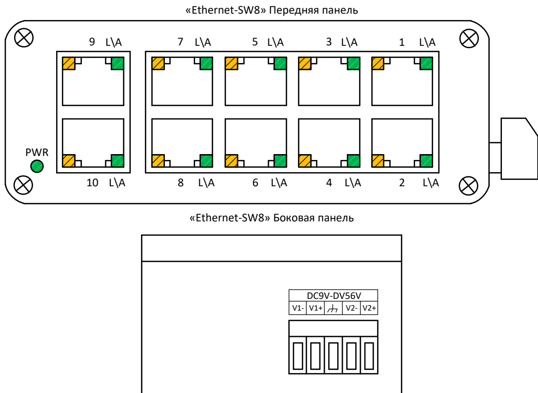
Рисунок 2.2.1 Внешний вид коммутатора
