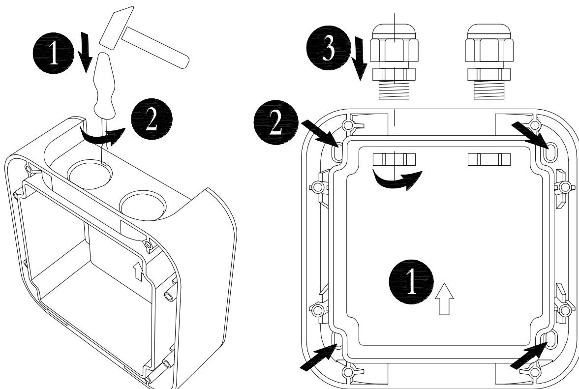
Рисунок 2.2.3.1 Основание ИПР
