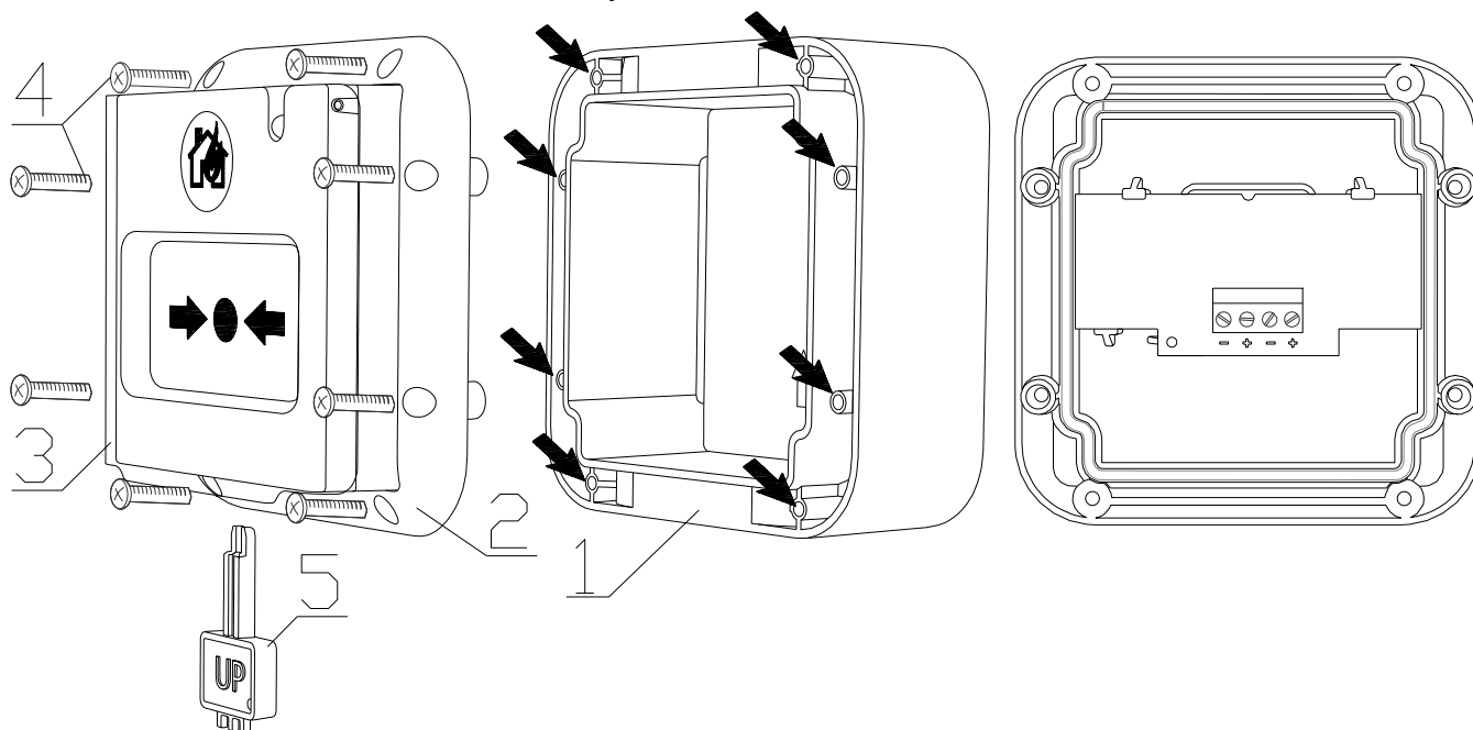
Рисунок 2.2.3.1 Основание ИПР
