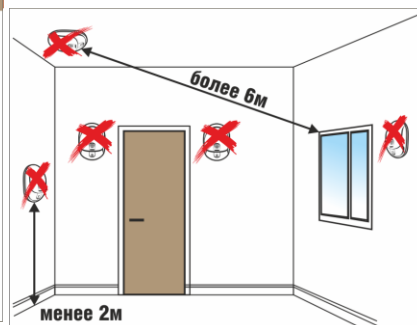
Рисунок 2.2.3.2.6 Нерекондуемые места установки извещателя
