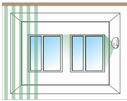
Рисунок 2.2.3.2.5 Установка извещателя между стеклом и занавесками (жалюзи)
