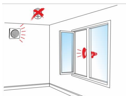
Рисунок 2.2.3.2.7 НЕрекомендуемые места установки извещателя
