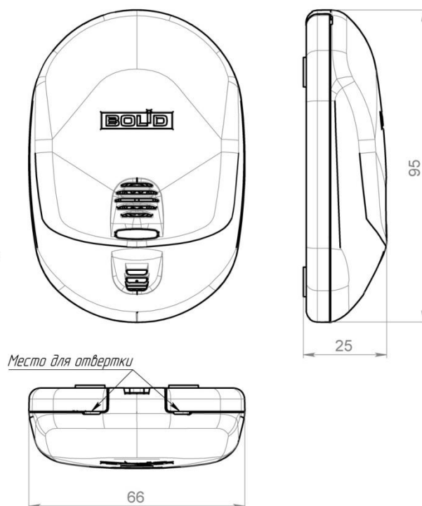
Рис.2.2.2.2. Габаритные размеры извещателя.
