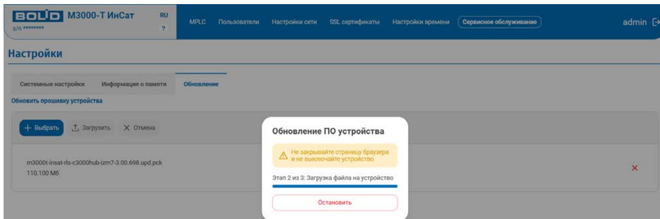
Рисунок 49, позиция 3. Обновление прошивки на устройстве через веб-конфигуратор. Окно загрузки файлов на устройство.
