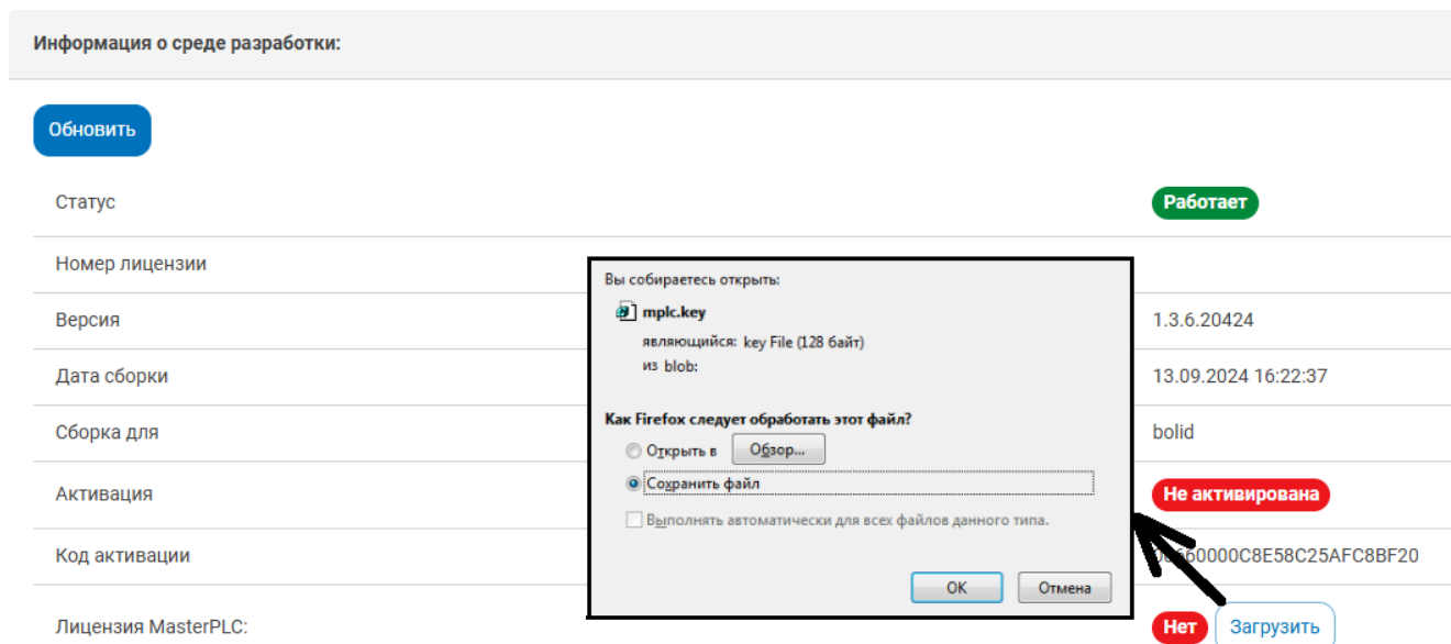
Рисунок 33. Диалоговое окно открытия файла лицензии
