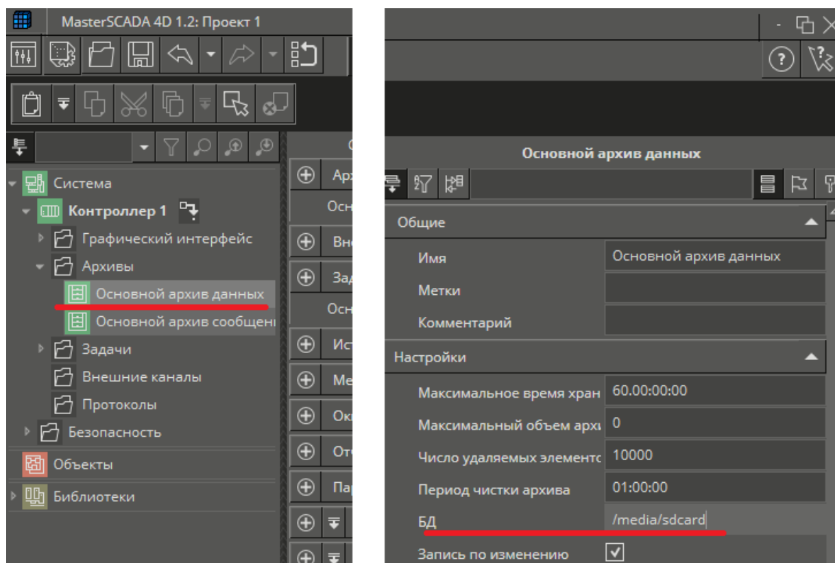
Рисунок 29.2. Фрагменты окна среды разработки MasterSCADA 4D с элементами настройки архива (дерево объектов слева и настройки архивирования справа). Архивирование производится по изменению на внешнюю SD-карту.
