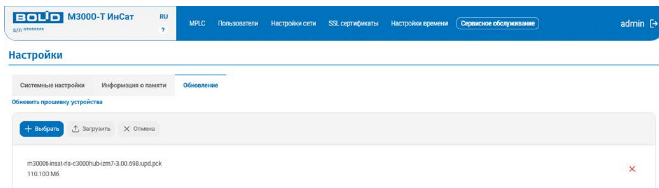
Рисунок 49, позиция 1. Страница «Сервисное обслуживание», вкладка «Обновление». Файл прошивки загружен в конвертер веб-конфигуратора ПЛК.
