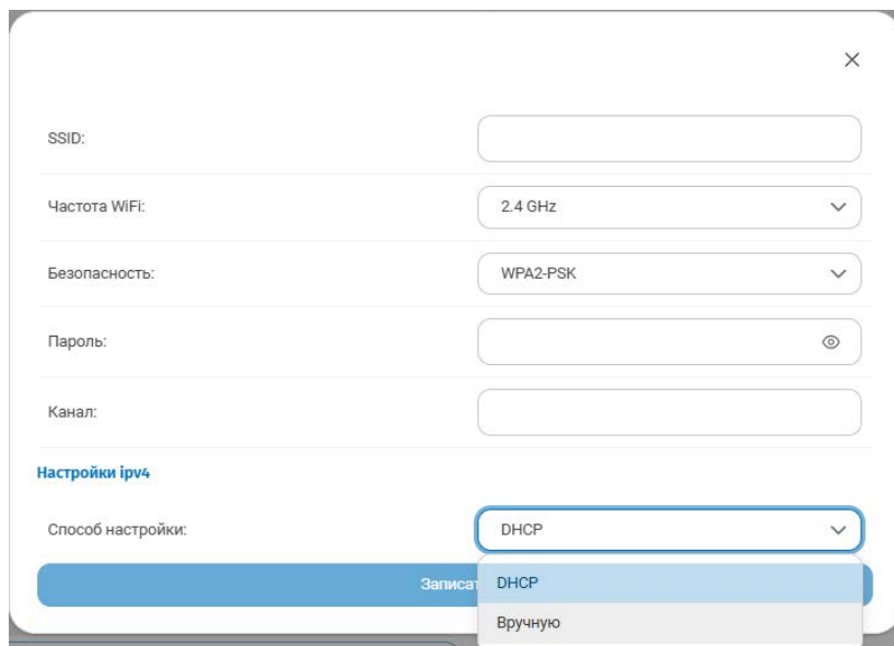
Рисунок 8, позиция 5. Настройки сети, вкладка "Wi-Fi". Ручное подключение к точке. Ручное выставление параметров подключения к Wi-Fi точке.
