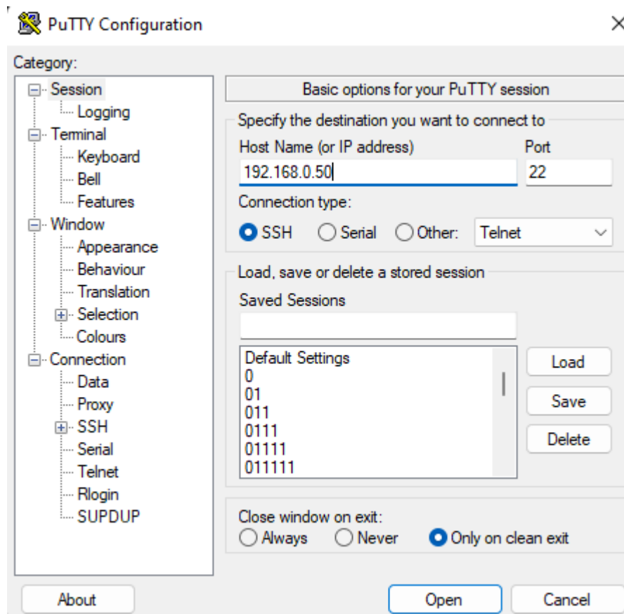
Рисунок 39. Ввод IP-адреса контроллера
