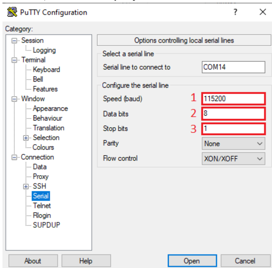
Рисунок 43. Установка параметров MicroUSB подключения
