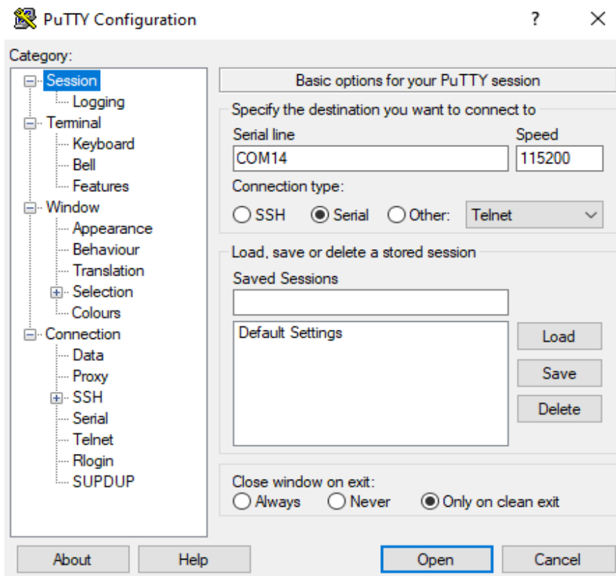
Рисунок 44. Установка параметров соединения
