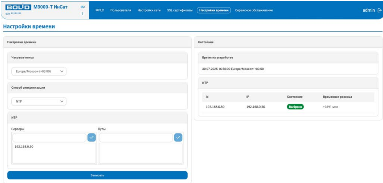
Рисунок 26.4. Страница настройки времени. Настройка NTP.
