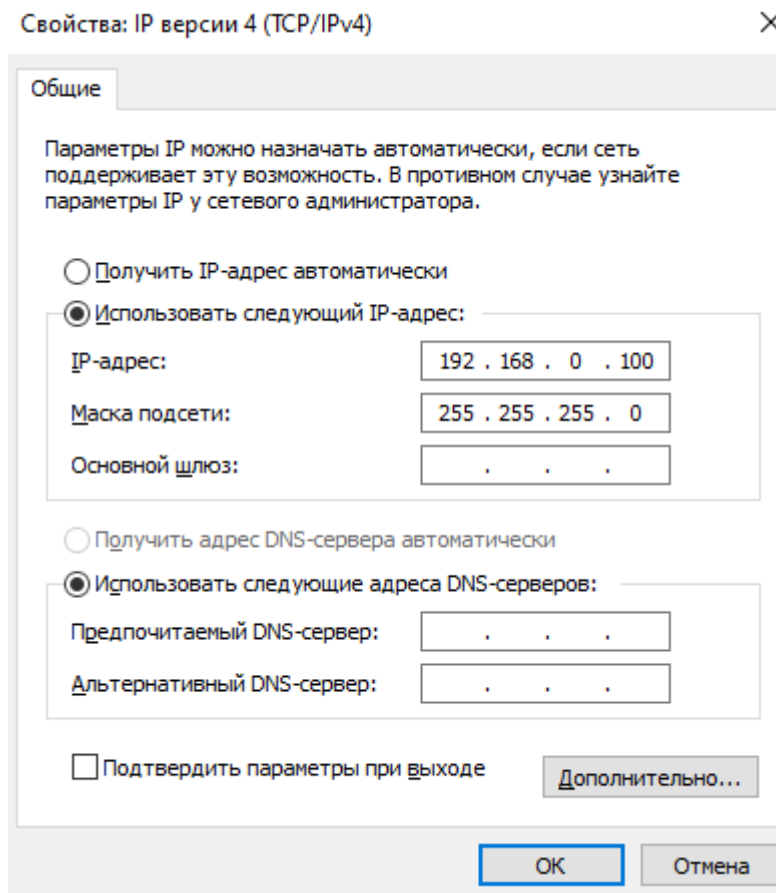
Рисунок 35. Сетевой адрес компьютера и маска подсети
