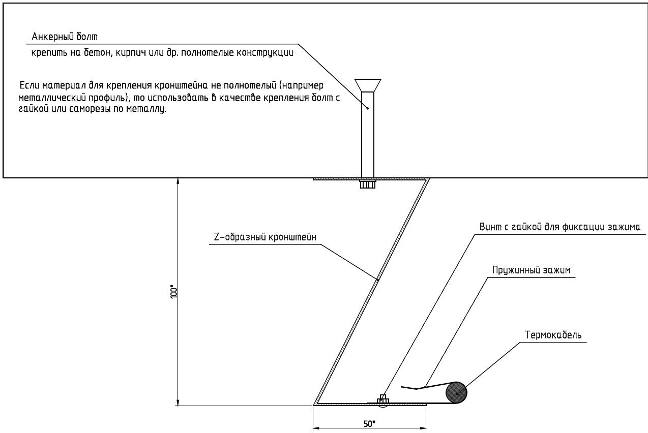
Рисунок 1. Чертеж МЭТ-01-01
