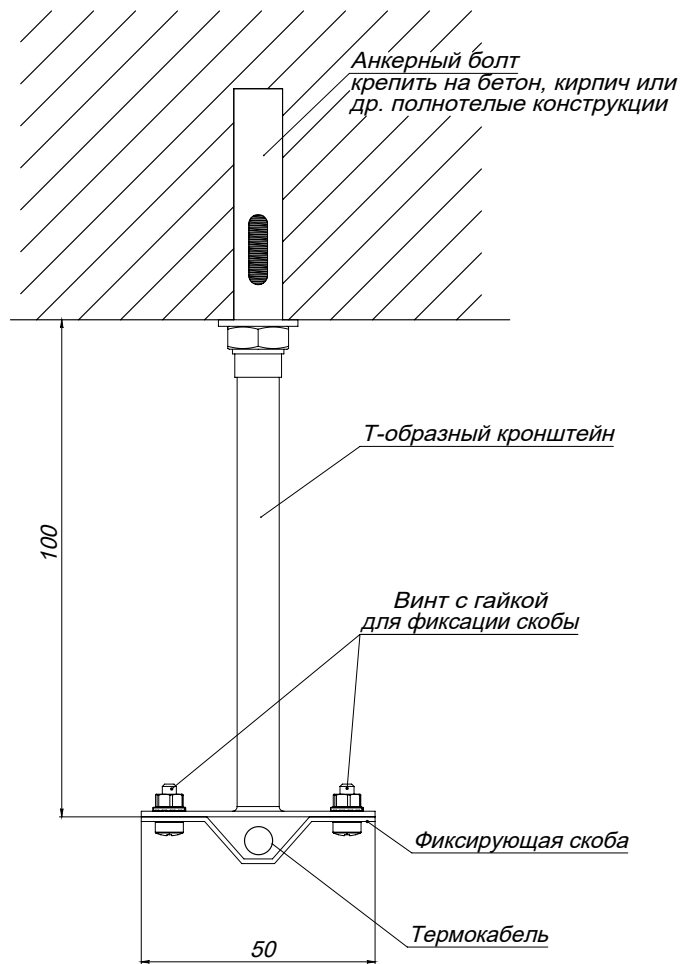
Рисунок 1. Чертеж МЭТ-01-02
