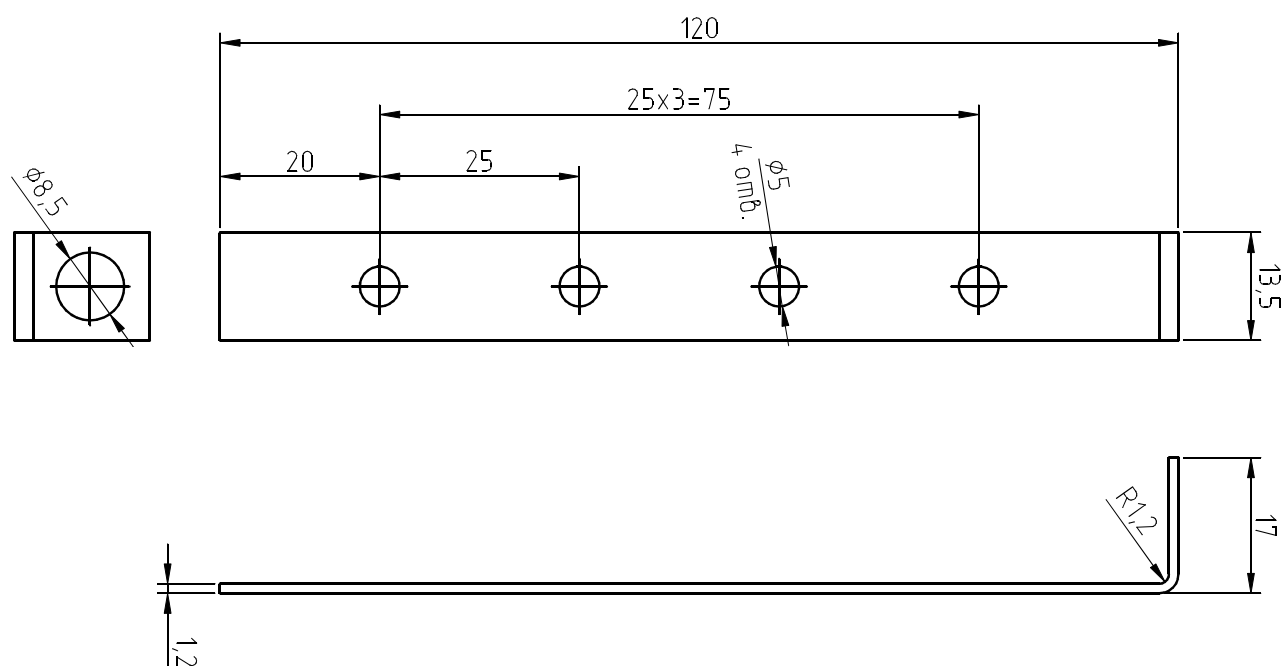
Рисунок 1. Чертеж МЭТ-01-03
