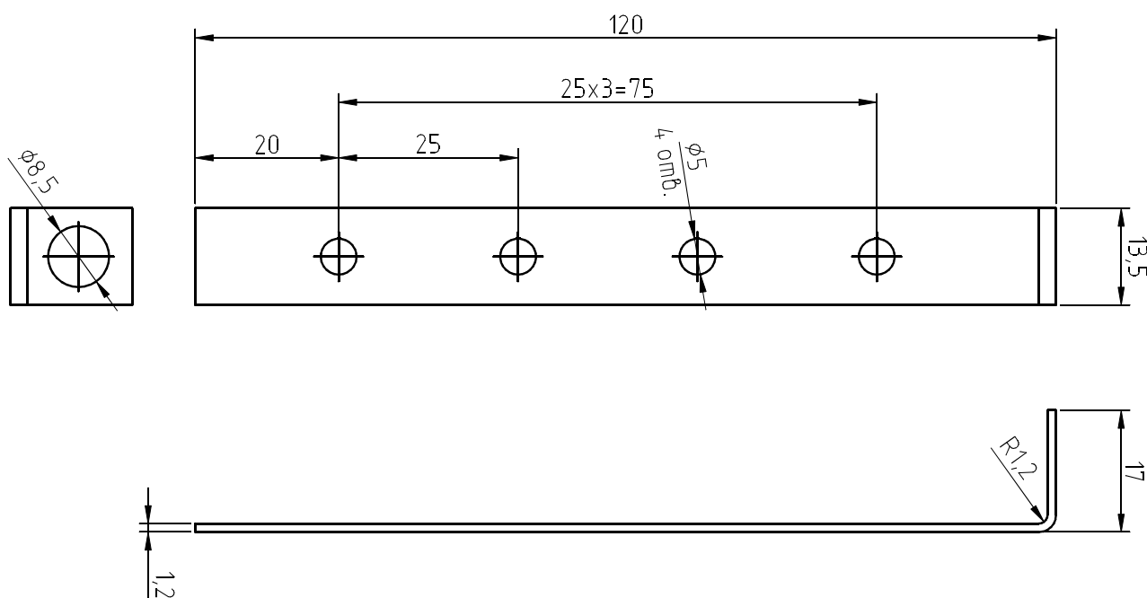
Рисунок 1. Чертеж МЭТ-01-03
