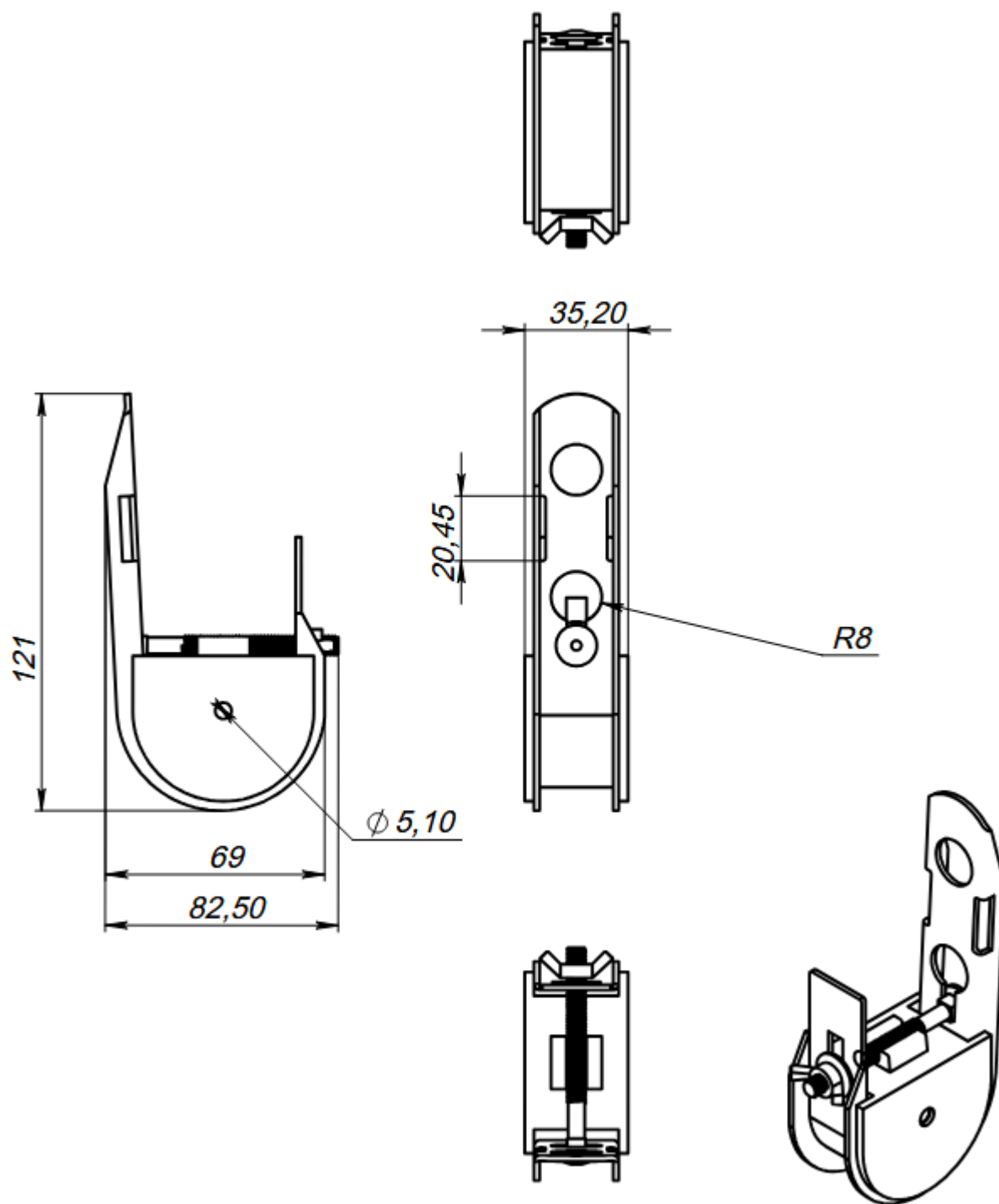
Рисунок 1. Чертёж МЭТ-01-05
