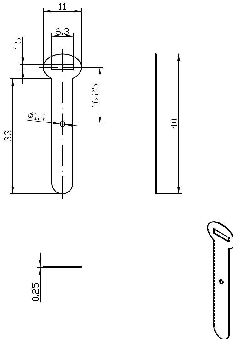
Рисунок 1. Чертёж МЭТ-03-02
