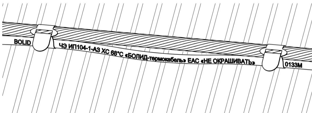
Рисунок 3. Пример размещения МЭТ-03-03. Крепление кабеля к несущему тросу.
