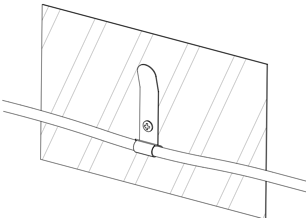
Рисунок 2. Пример размещения МЭТ-03-03. Крепление кабеля к несущей поверхности.
