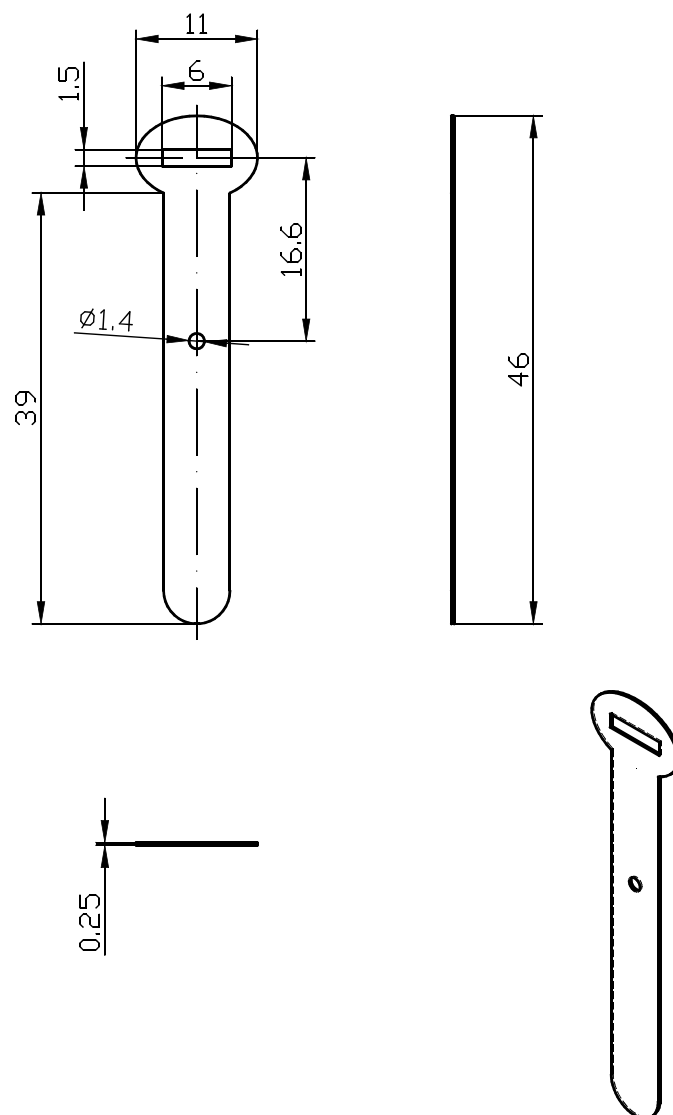
Рисунок 1. Чертёж МЭТ-03-03
