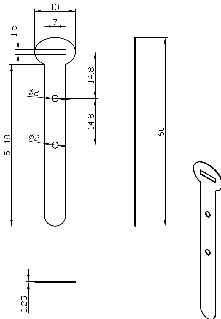
Рисунок 1. Чертёж МЭТ-03-04
