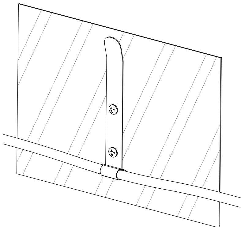
Рисунок 2. Пример размещения МЭТ-03-04. Крепление кабеля к несущей поверхности.
