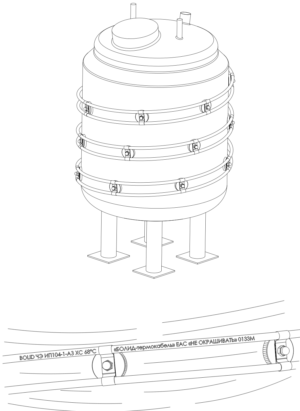
Рисунок 2. Пример размещения МЭТ-05-02
