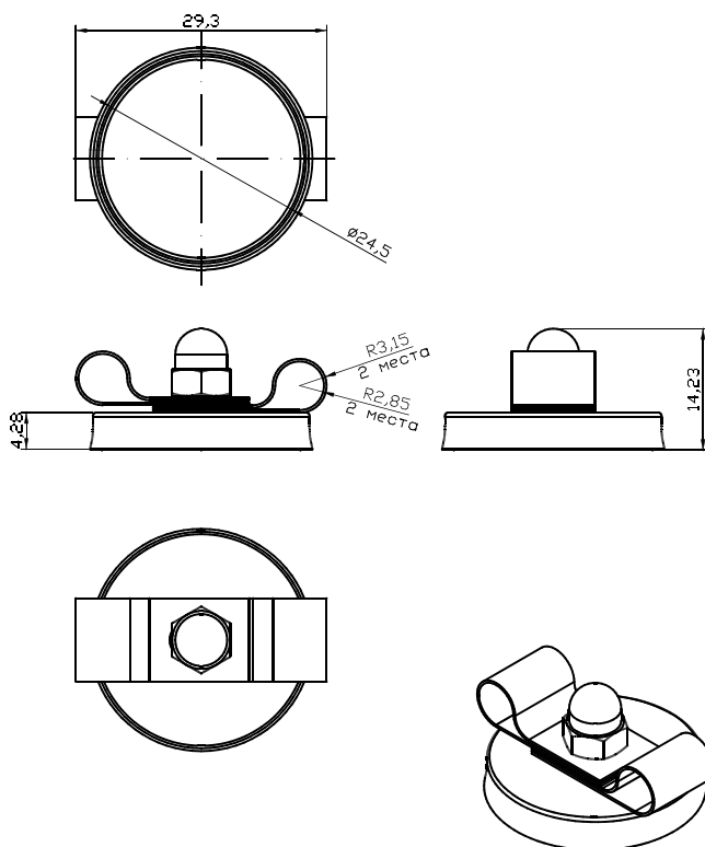
Рисунок 1. Чертёж МЭТ-05-02
