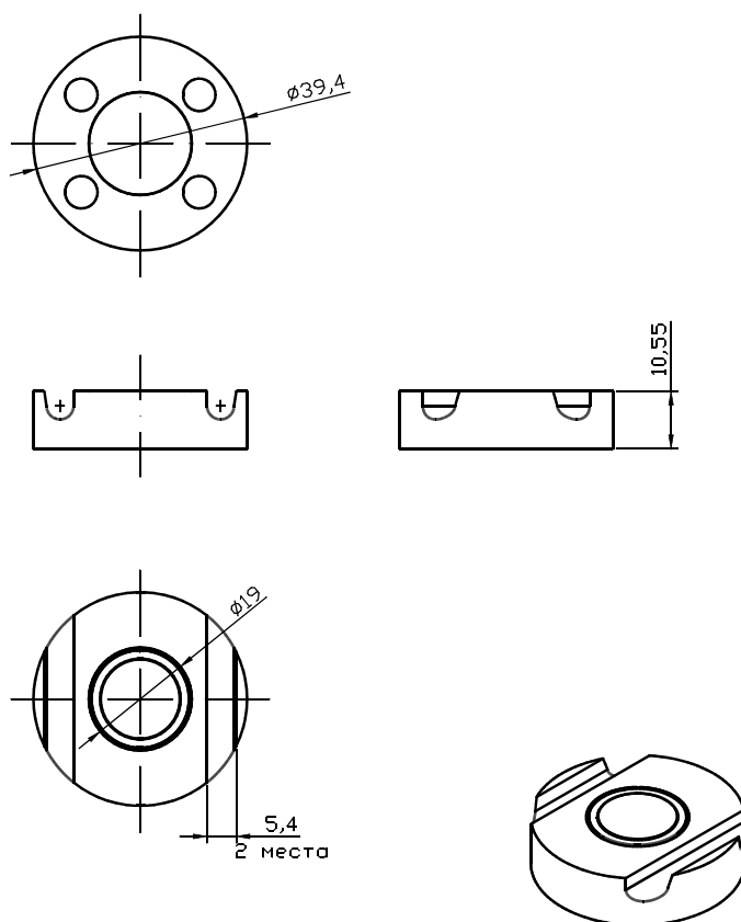
Рисунок 1. Чертёж МЭТ-05-03
