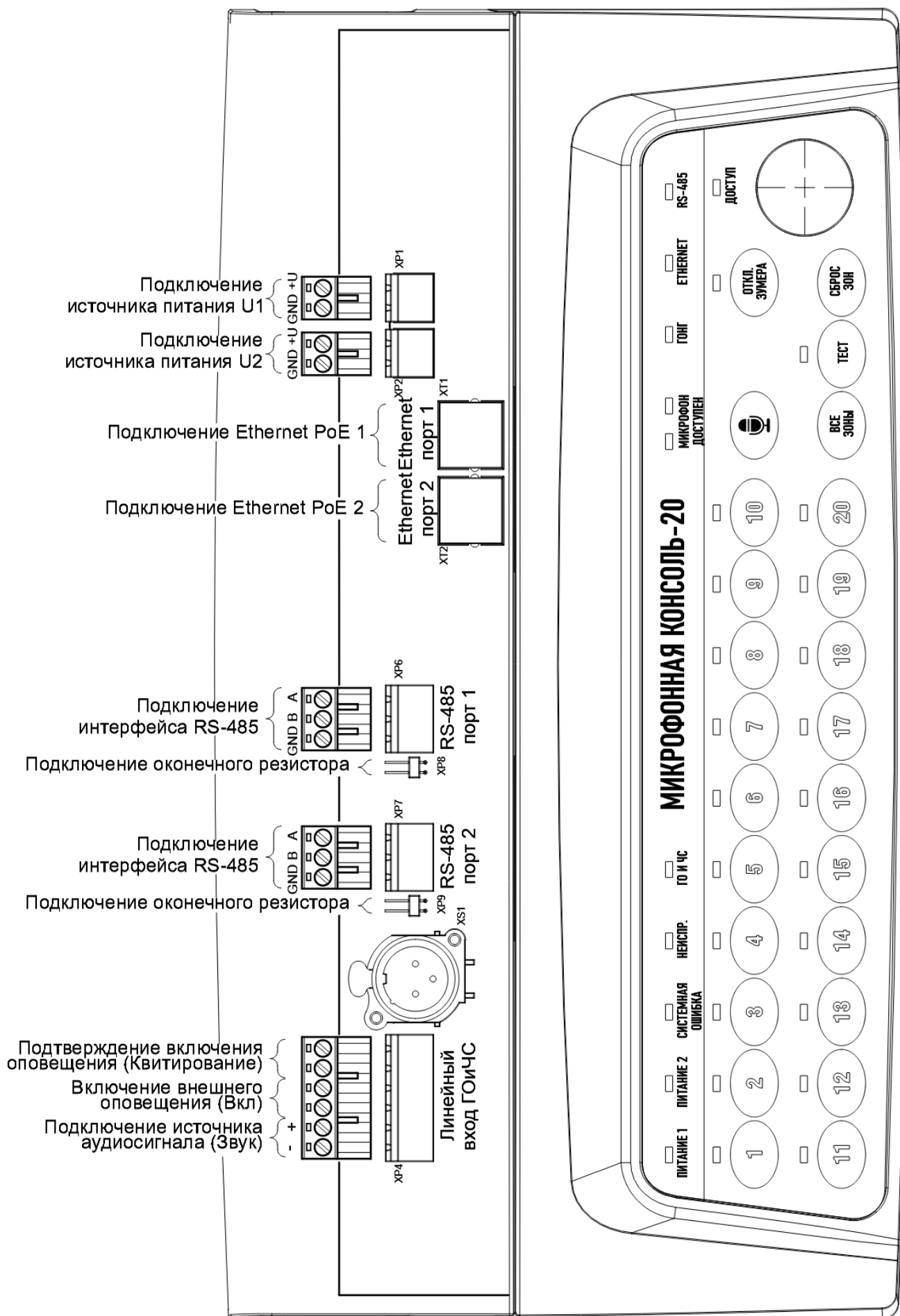
Рисунок 2.2.3. Схема подключения консоли.
