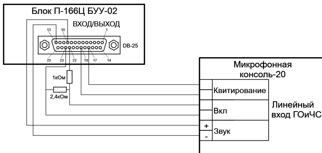
Рисунок 1.4.3. Схема подключения блока управления П-166Ц БУУ-02.
