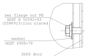
SECTION D-D
