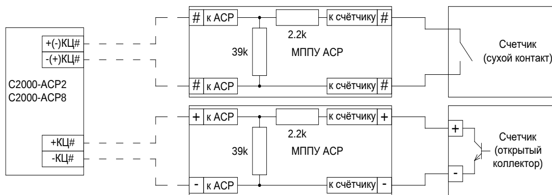
Рисунок 2.2.2 Схема подключения.
