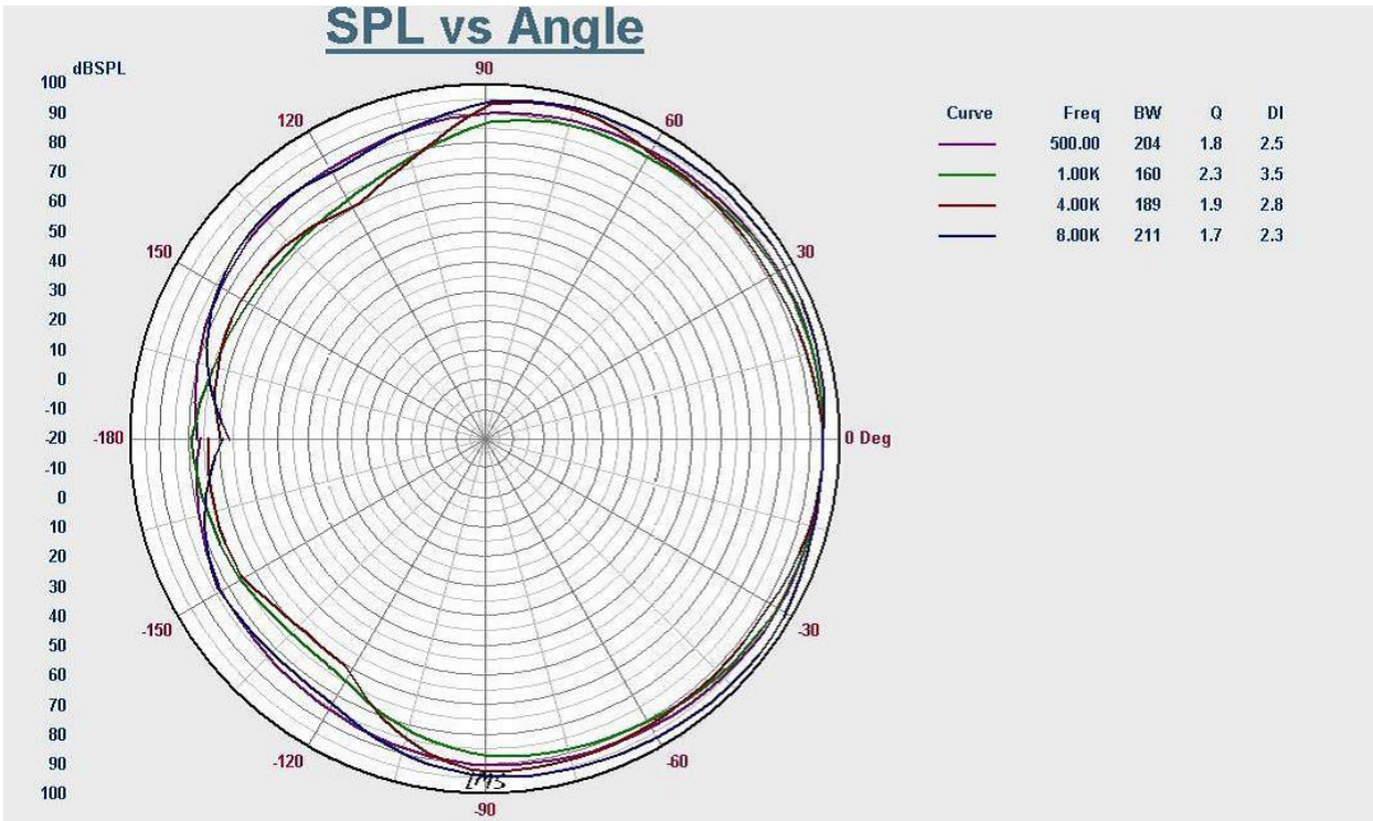
Диаграмма направленности
