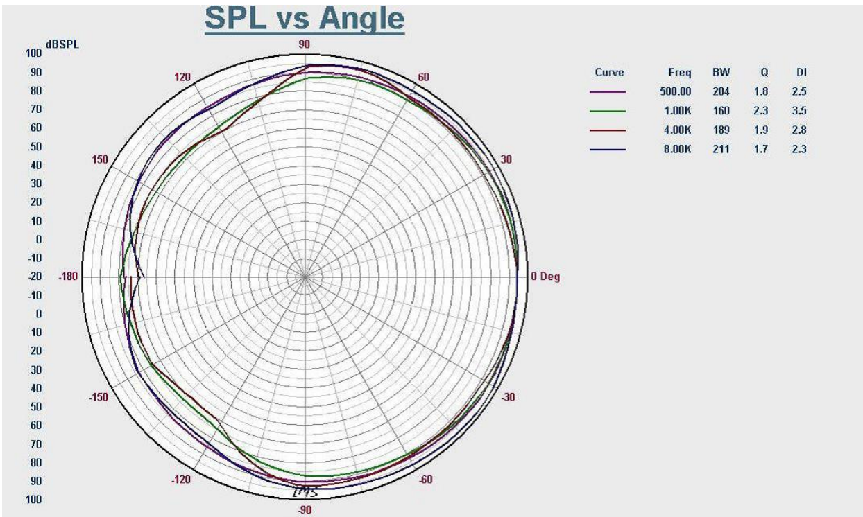
Диаграмма направленности
