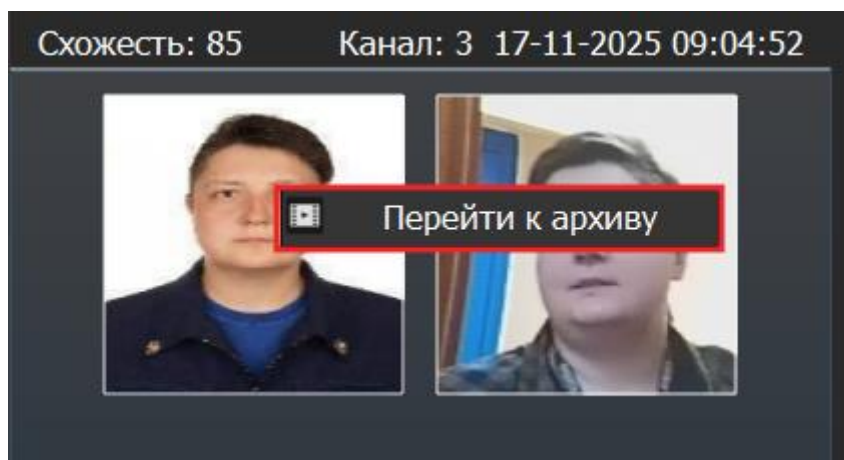
Рисунок 9.12 – Результаты поиска
