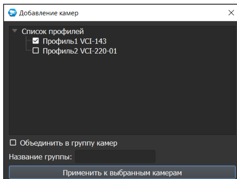
Рисунок 4.25 – Настройка профиля
