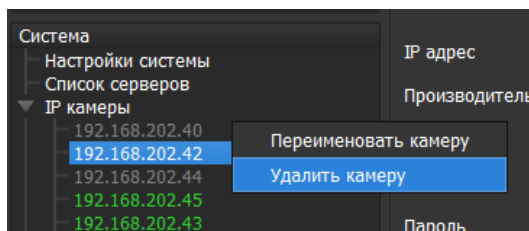
Рисунок 6.7 – Удаление видеокamеры
