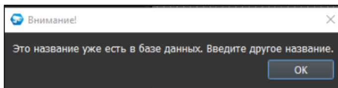
Рисунок 7.56 – Окно сообщения
