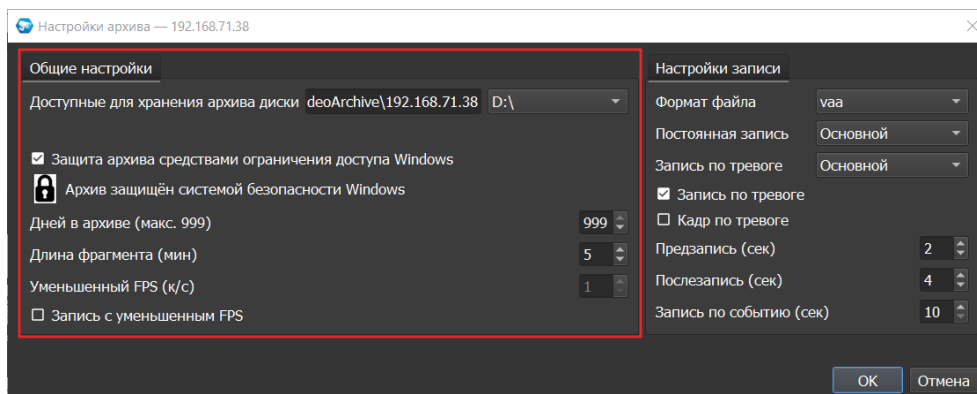
Рисунок 8.9 – Общие настройки
