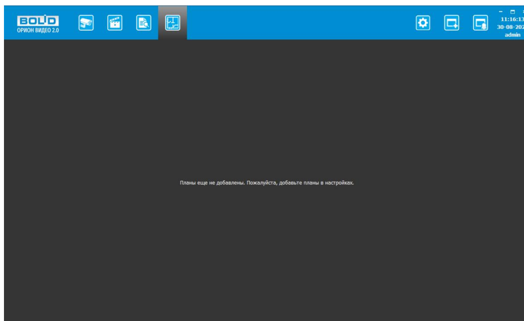
Рисунок 11.14 – Планы помещений
