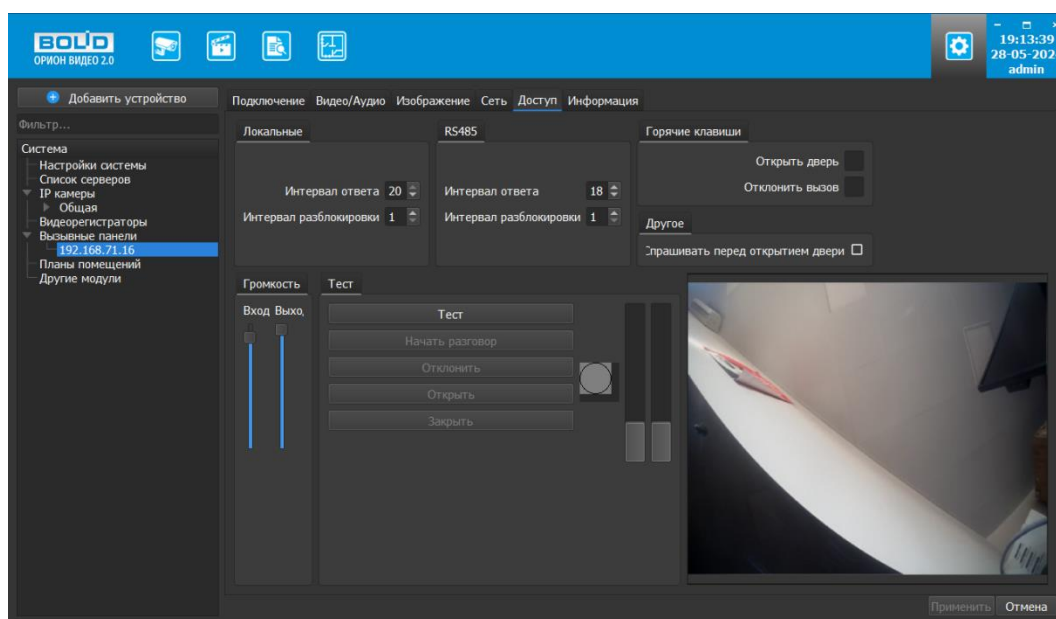
Рисунок 6.83 – Вкладка «Доступ»
