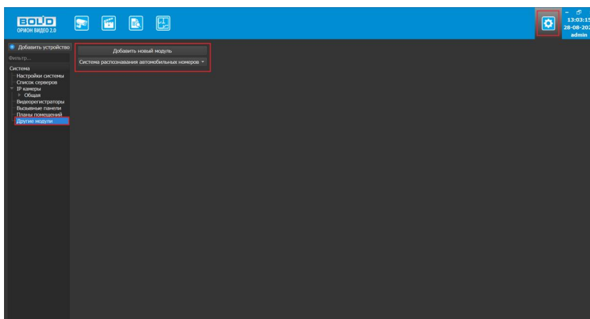
Рисунок 12.2 – Другие модули
