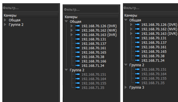
Рисунок 7.4 – Список устройств
