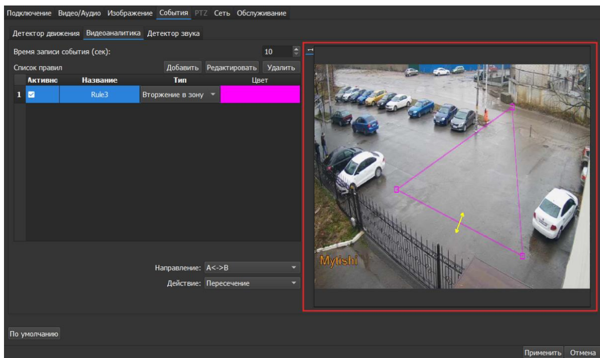
Рисунок 6.21 – Настройка видеоаналитики
