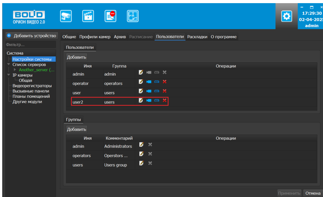
Рисунок 4.44 – Импорт пользователей
