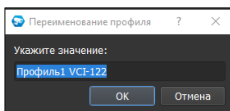
Рисунок 4.16 – Переименовать профиль
