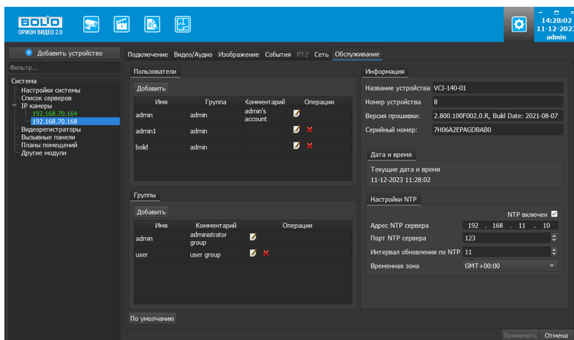
Рисунок 5.17 – Вкладка «Обслуживание»
