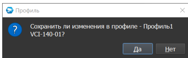
Рисунок 4.18 – Окно подтверждения
