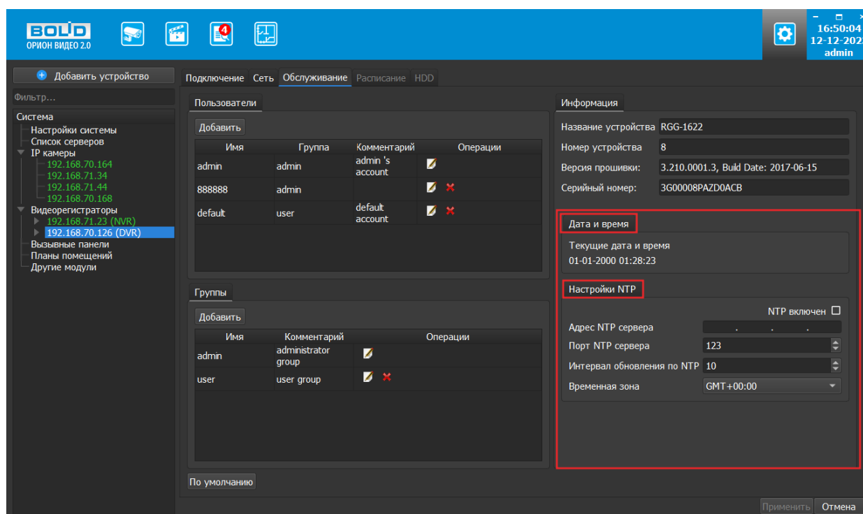
Рисунок 6.62 – Вкладка «Обслуживание»
