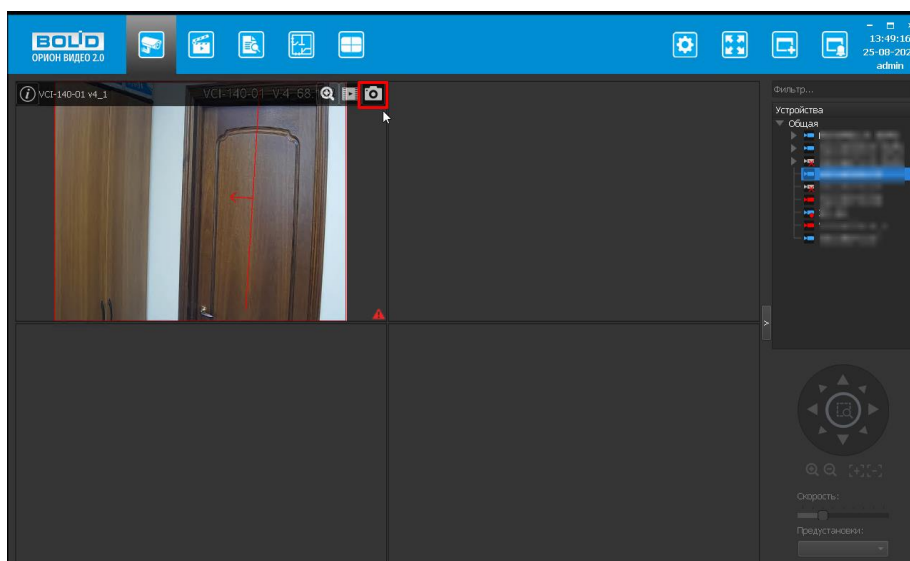
Рисунок 7.35 – Создание кадра
