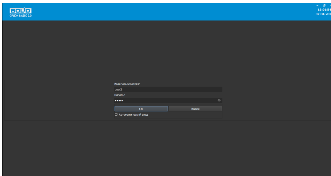
Рисунок 4.45 – Вход
