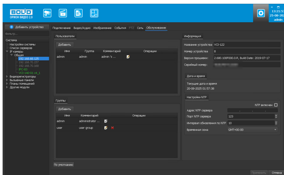
Рисунок 6.45 – Вкладка «Обслуживание»
