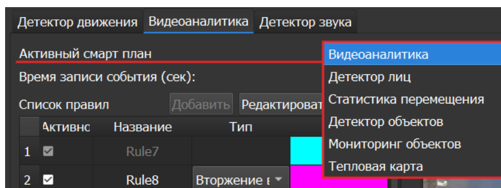
Рисунок 6.30 – Выбор смарт-плана
