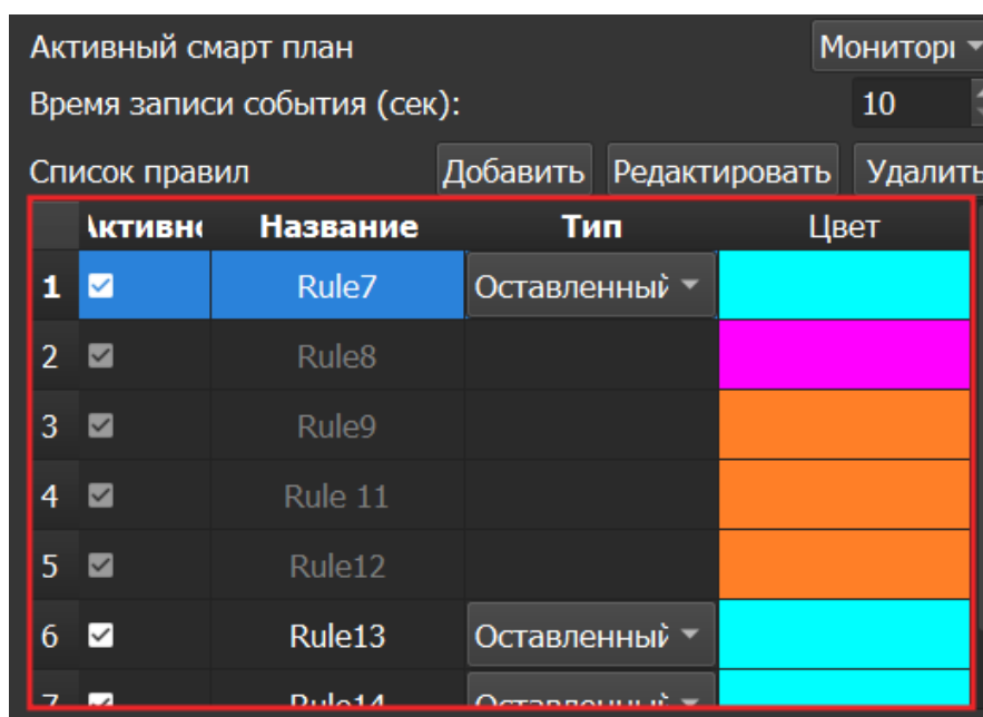
Рисунок 6.29 – Список правил
