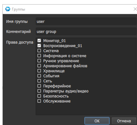
Рисунок 5.25 – Добавление групп
