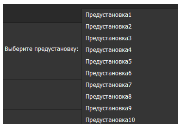
Рисунок 6.16 – Выбор предустановки
