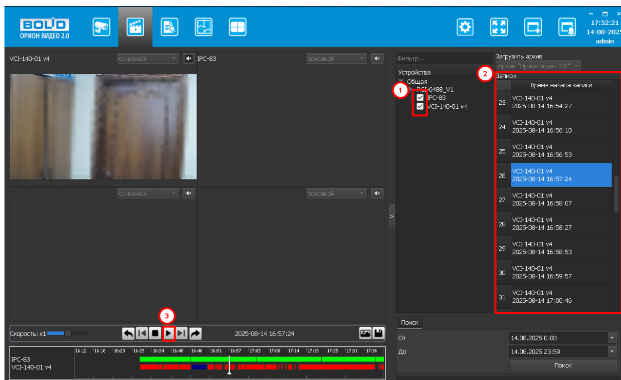
Рисунок 8.13 – Воспроизведение записи
