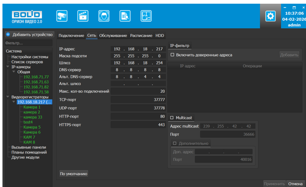
Рисунок 6.60 – Вкладка «Сеть»
