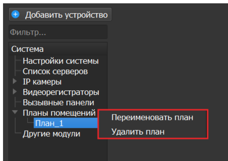
Рисунок 11.4 – Контекстное меню
