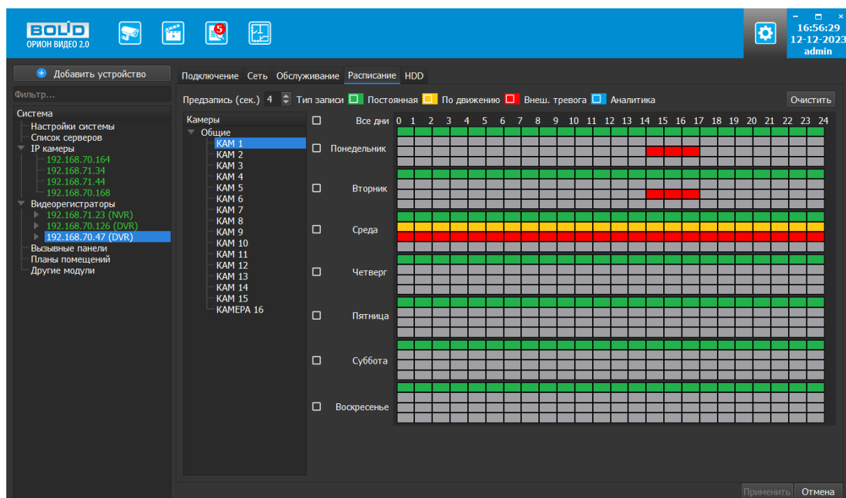
Рисунок 6.67 – Вкладка «Расписание»
