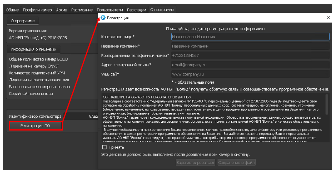
Рисунок 4.32 – Регистрация ПО
