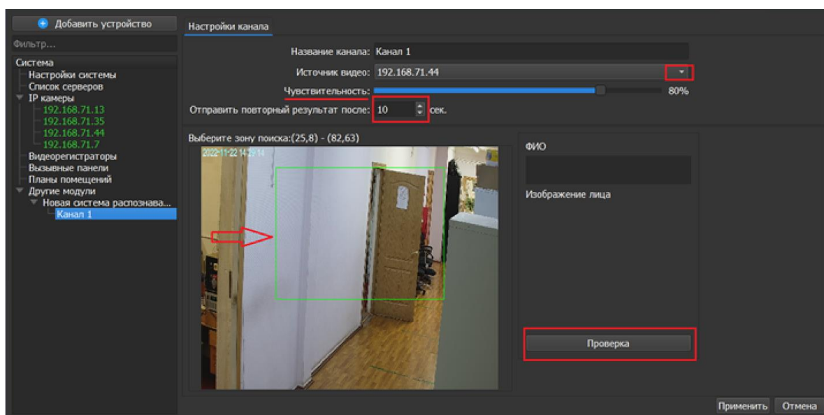
Рисунок 12.12 – Настройка
