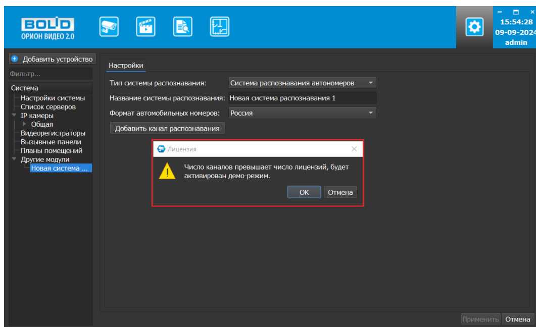
Рисунок 12.9 – Настройка
