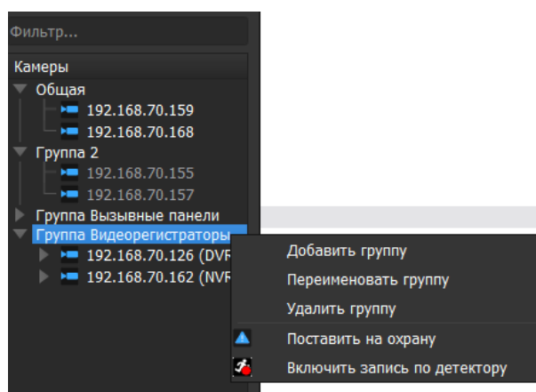
Рисунок 7.11 – Список устройств
