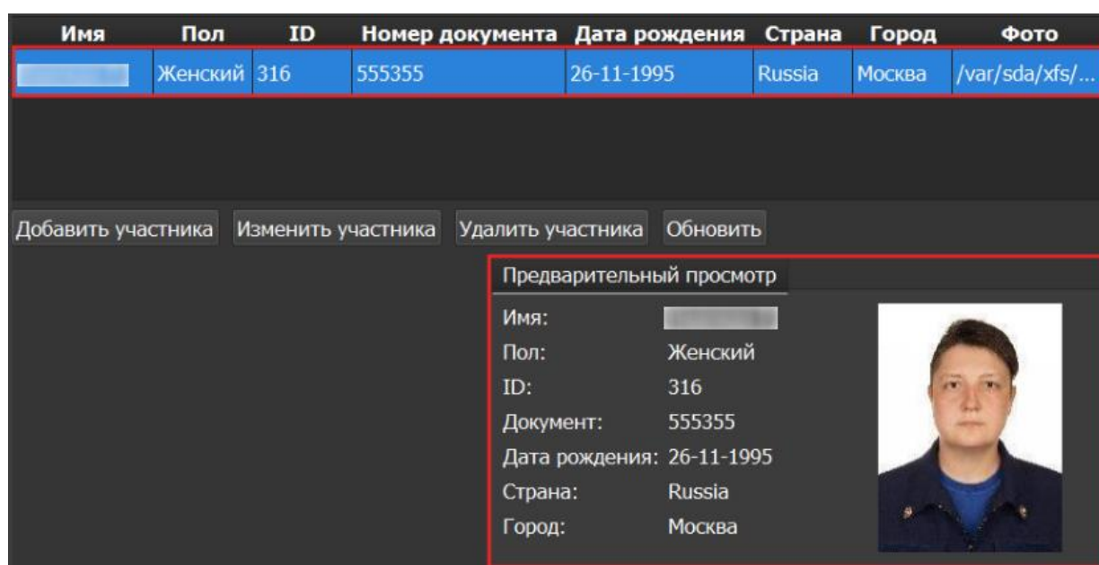
Рисунок 9.31 – Предварительный просмотр
