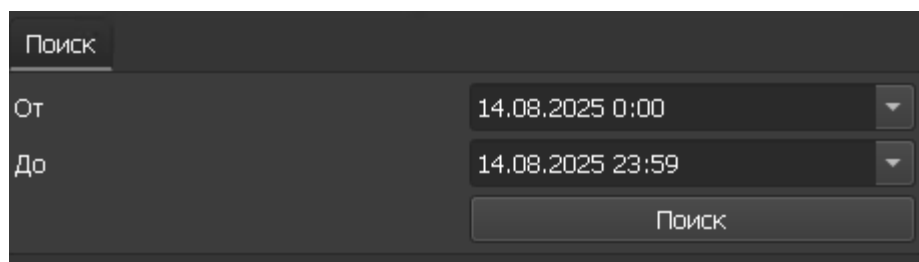
Рисунок 8.15 – Поиск
