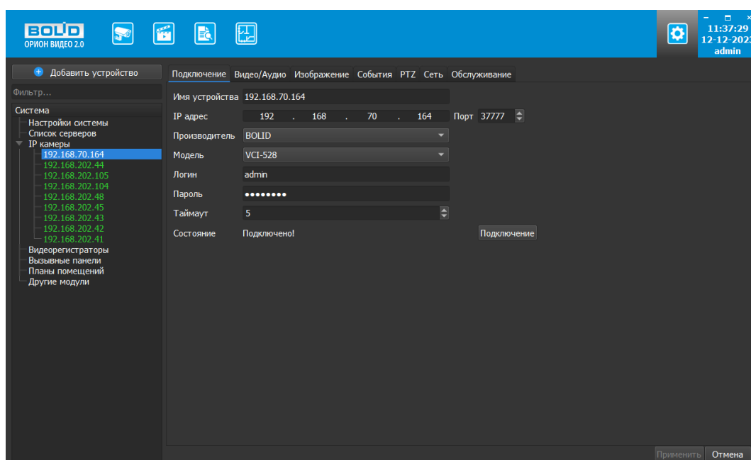
Рисунок 6.9 – Вкладка «Подключение»
