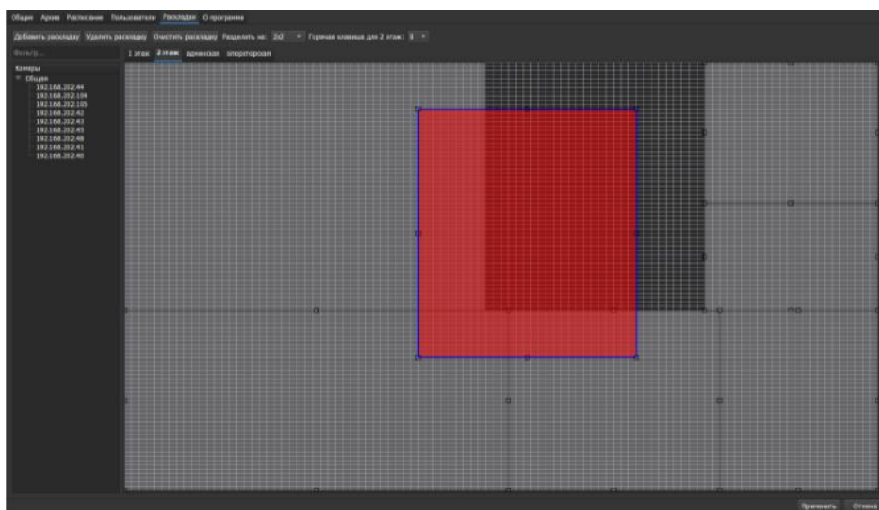
Рисунок 7.49 – Создание раскладки
