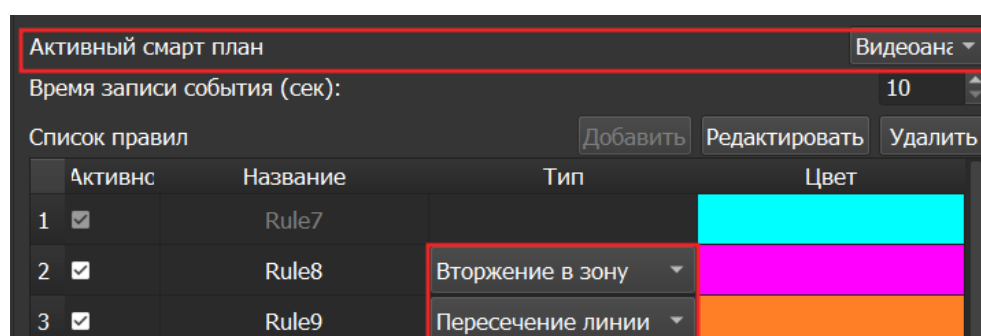
Рисунок 6.31 – Смарт-план «Видеоаналитика»
