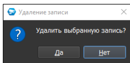
Рисунок 5.22 – Подтверждение удаления
