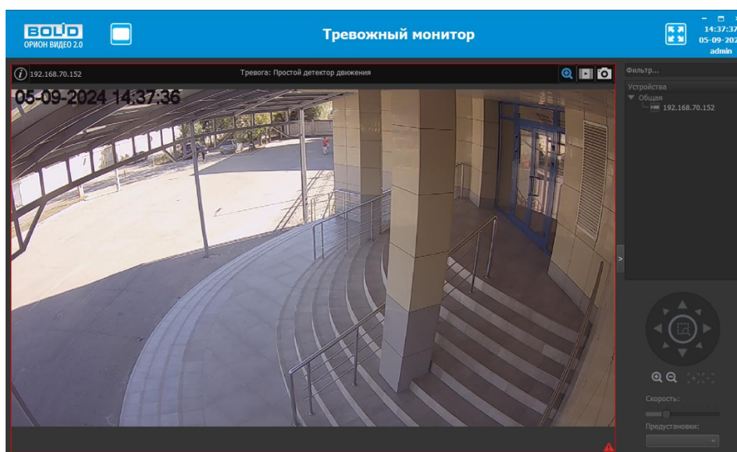
Рисунок 7.75 – Тревожный монитор
