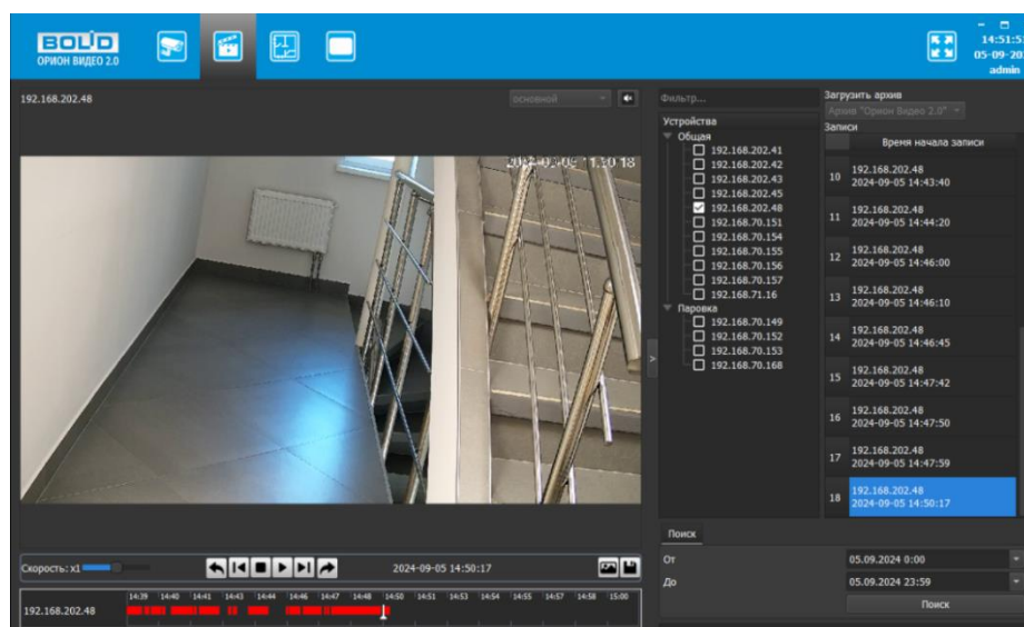
Рисунок 7.81 – Просмотр архива
