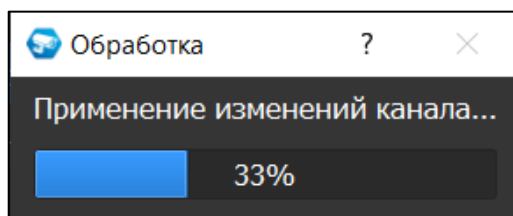
Рисунок 9.28 – Окно обработки
