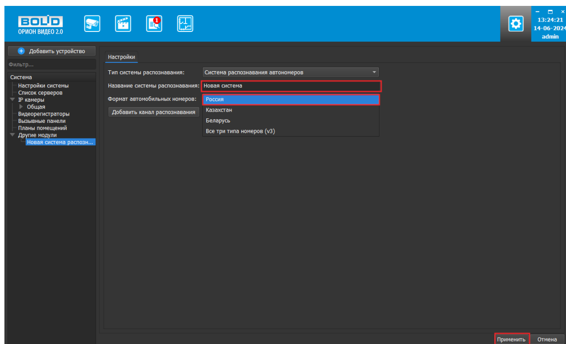
Рисунок 12.4 – Настройка модуля
