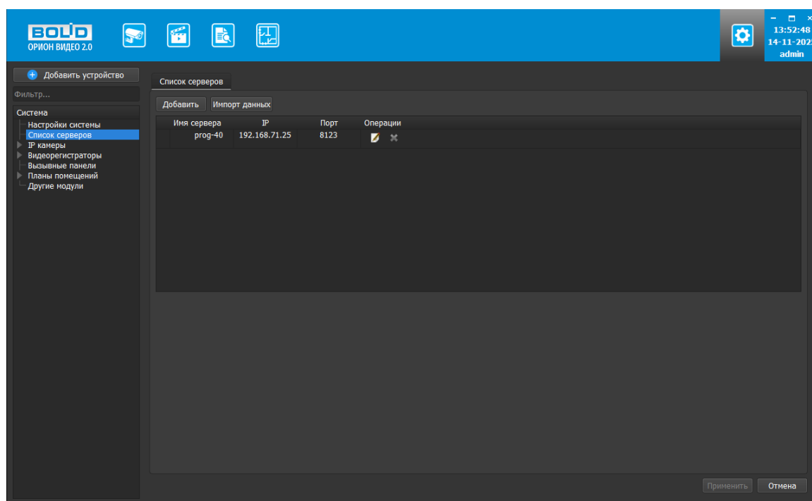
Рисунок 4.33 – Список серверов
