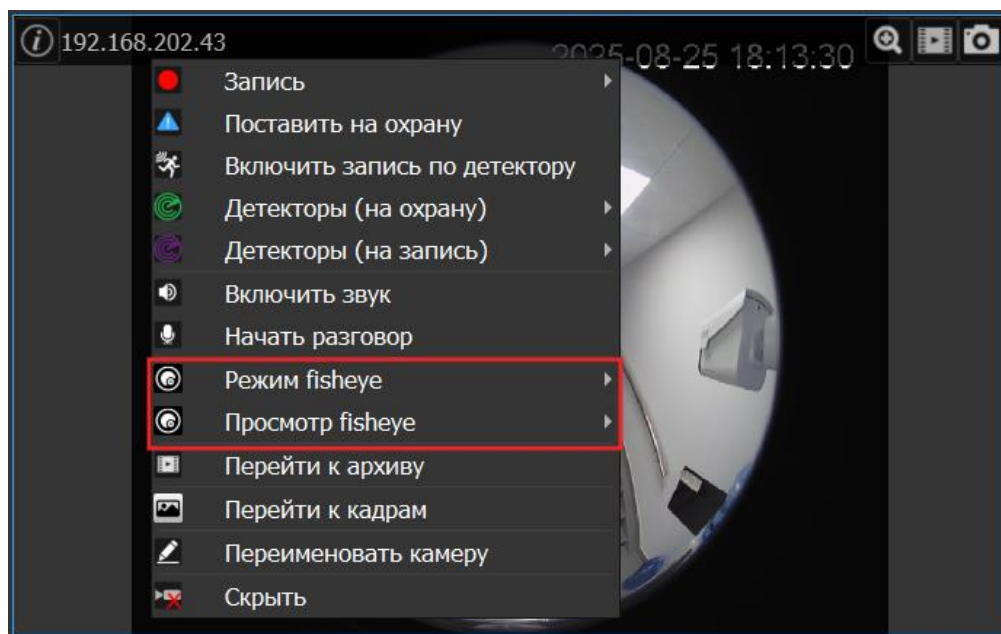
Рисунок 7.24 – Контекстное меню
