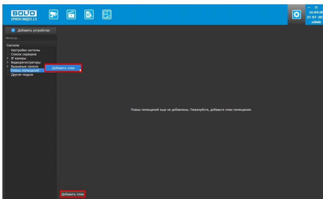
Рисунок 11.2 – Добавление плана
