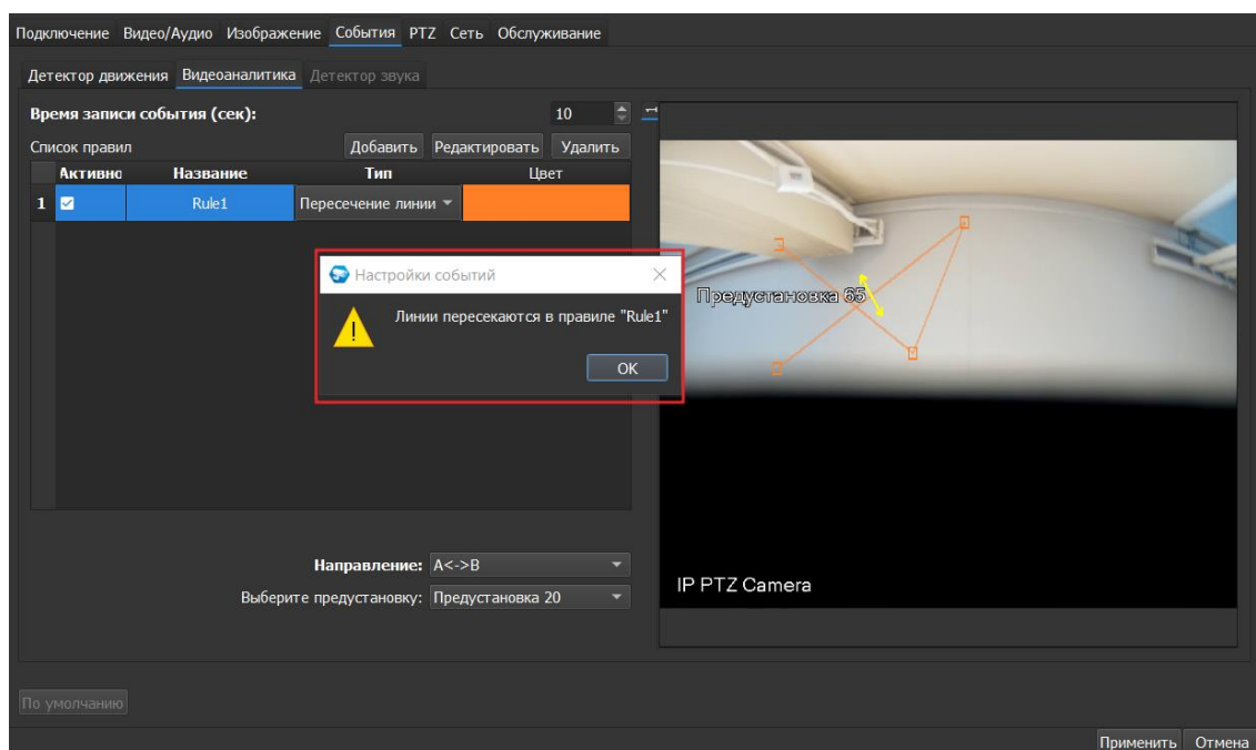
Рисунок 6.23 – Настройка видеоаналитики
