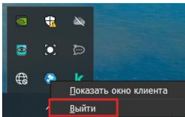
Рисунок 2.26 – Контекстное меню
