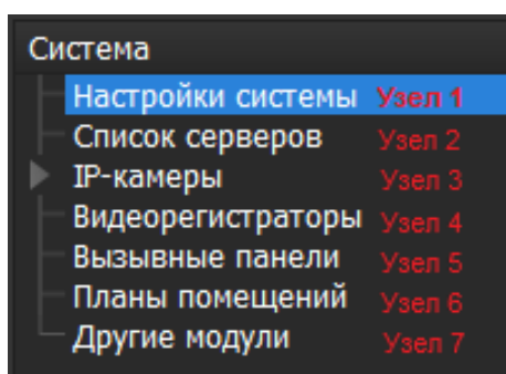
Рисунок 12.1 – Дерево системы
