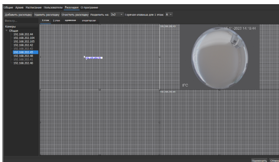
Рисунок 7.50 – Создание раскладки
