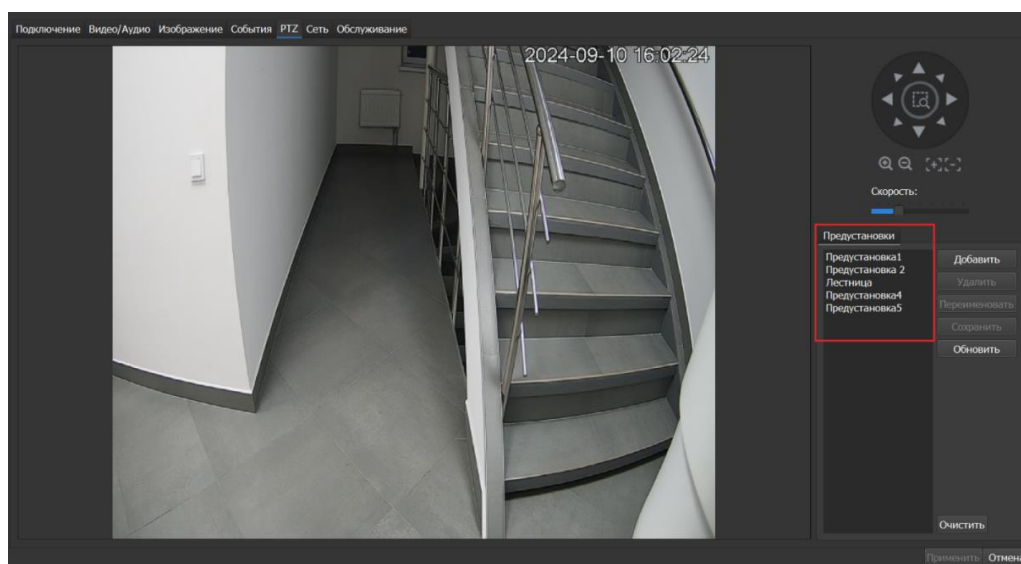
Рисунок 6.37 – Настройка PTZ
