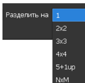
Рисунок 7.44 – Список раскладок
