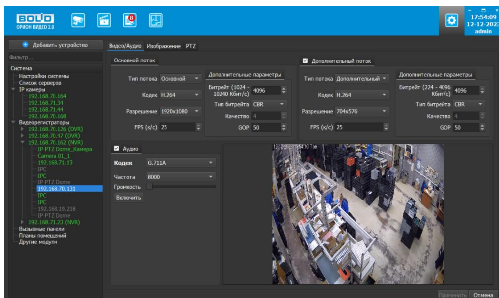
Рисунок 6.69 – Вкладка «Видео/Аудио»
