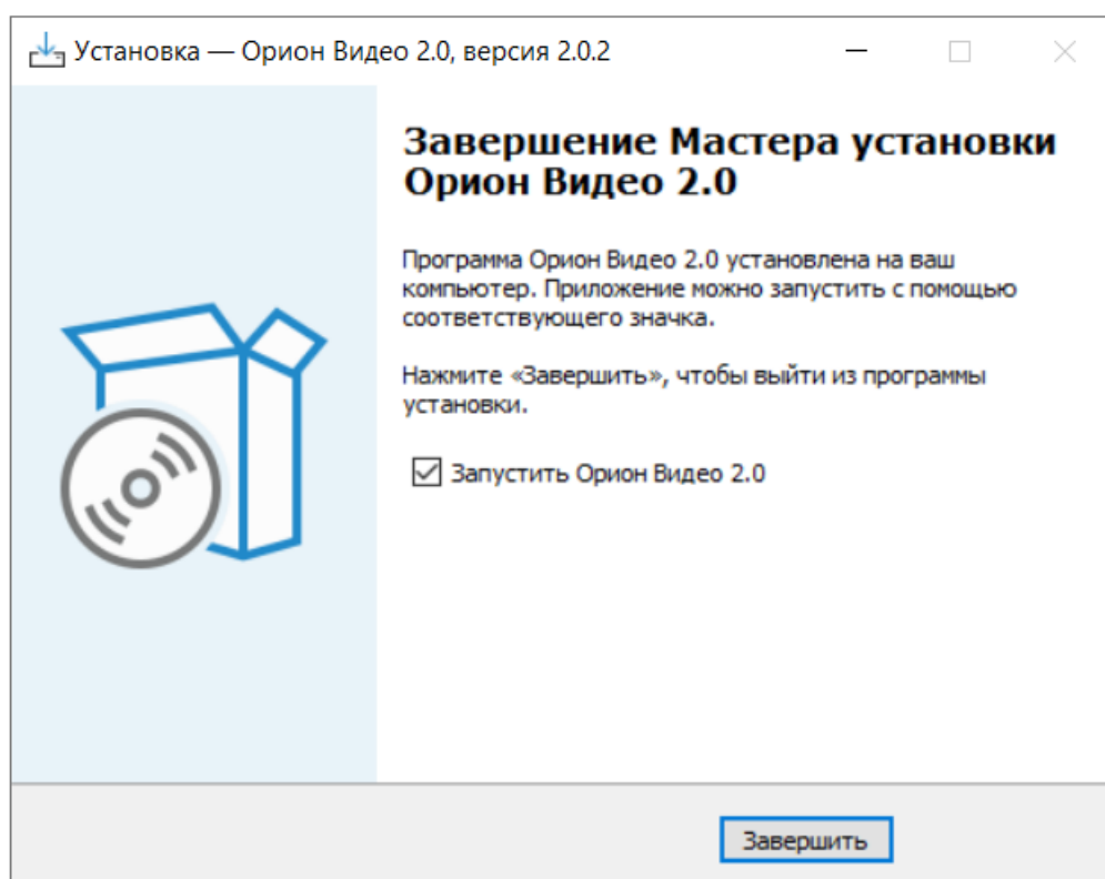
Рисунок 2.13 – Завершение установки
