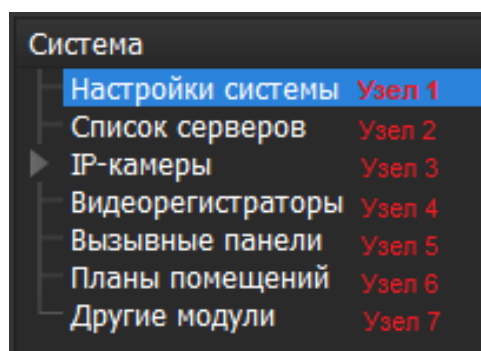
Рисунок 6.1 – Дерево системы
