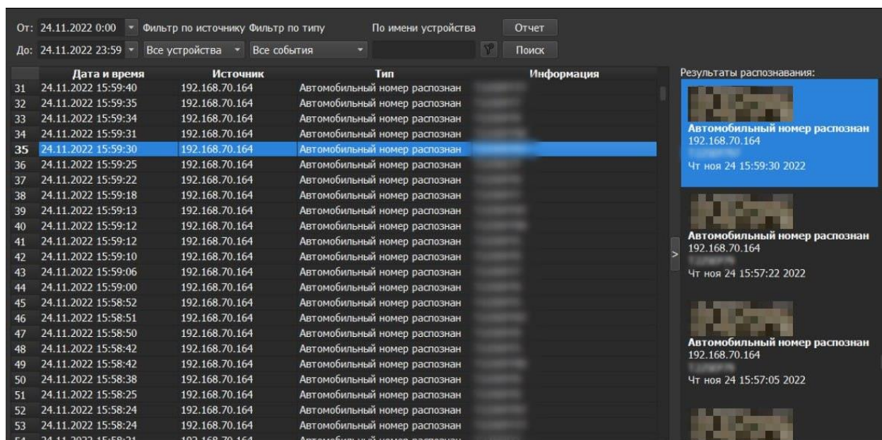
Рисунок 12.10 – Просмотр
