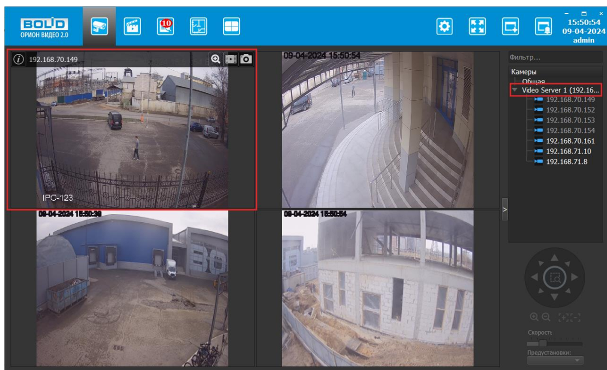
Рисунок 2.31 – Просмотр видео
