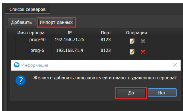
Рисунок 4.43 – Подтверждение импорта
