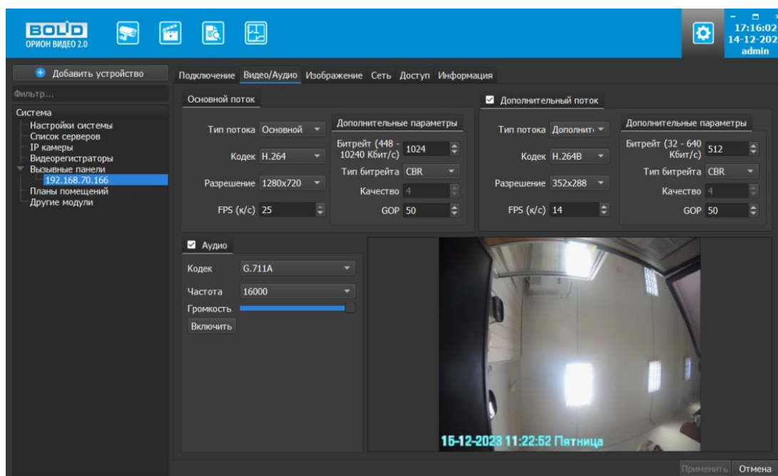
Рисунок 6.80 – Вкладка «Видео/Аудио»
