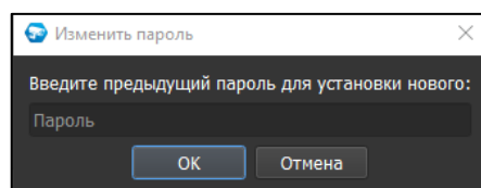
Рисунок 5.21 – Изменение пароля
