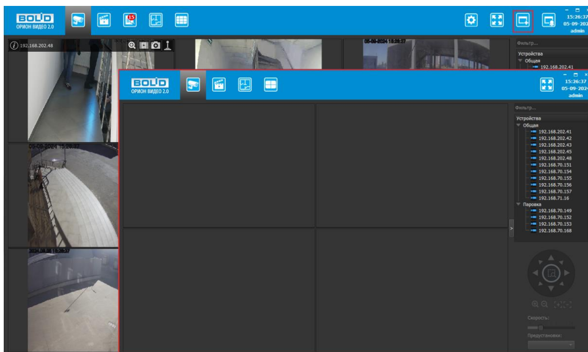
Рисунок 7.66 – Дополнительное окно
