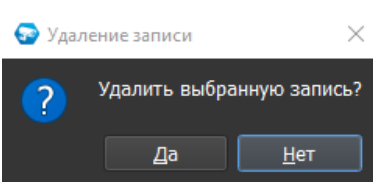
Рисунок 5.26 – Окно подтверждения
