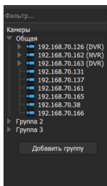
Рисунок 7.3 – Добавление группы
