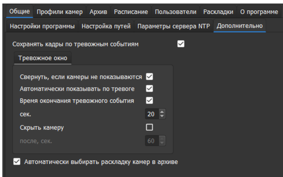
Рисунок 4.12 – Подкладка «Дополнительно»
