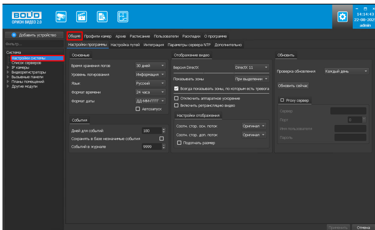
Рисунок 4.2 – Вкладка «Общие»
