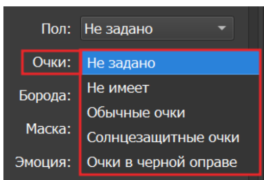
Рисунок 9.17 – Атрибут «Очки»
