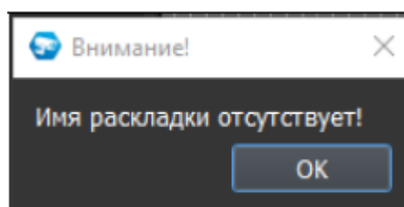
Рисунок 7.55 – Переименовать раскладку
