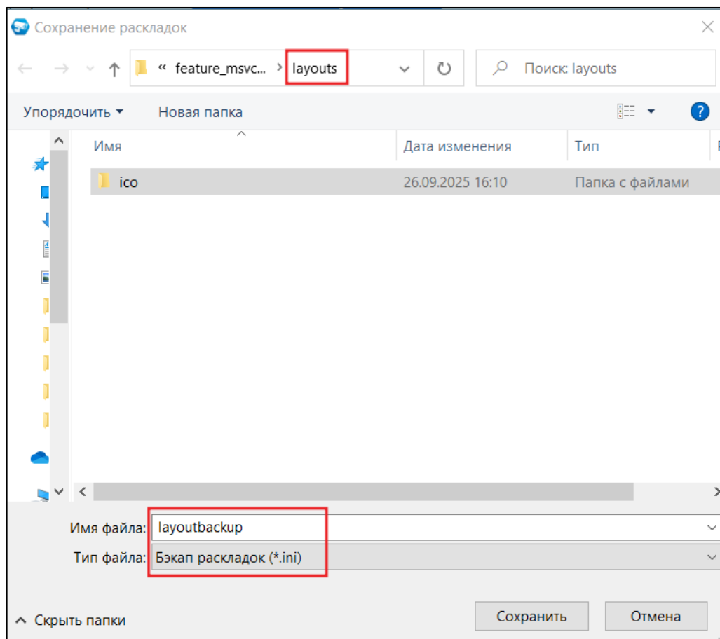
Рисунок 7.60 – Сохранение раскладок
