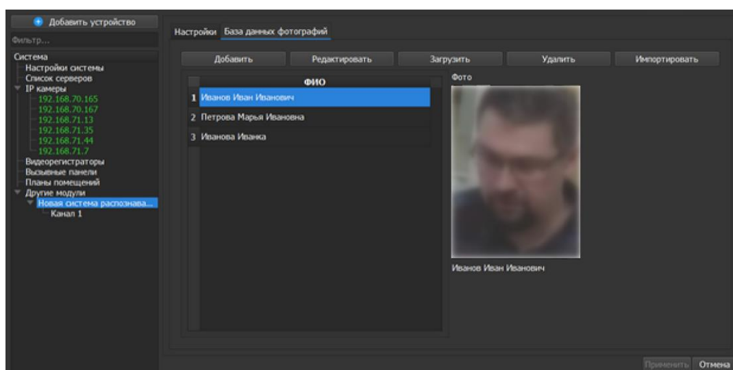
Рисунок 12.17 – Добавление
