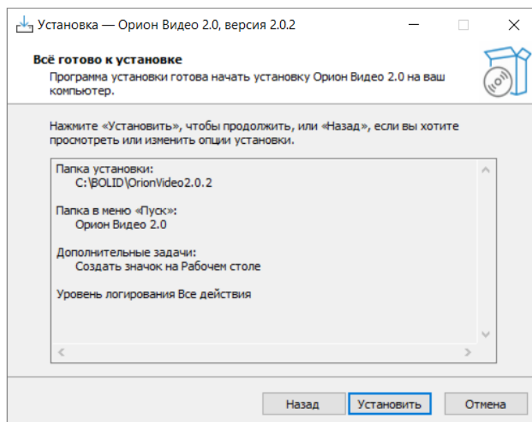
Рисунок 2.11 – Подтверждение установки
