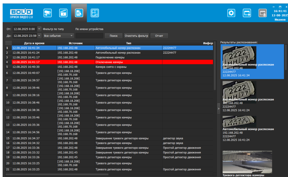
Рисунок 10.11 – Панель событий
