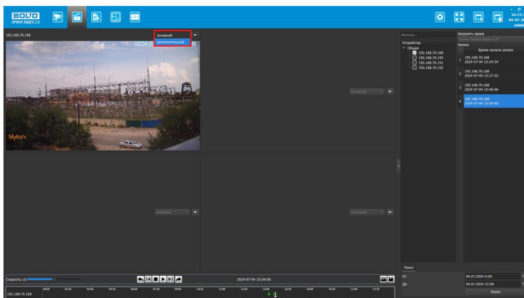
Рисунок 8.17 – Выбор потока
