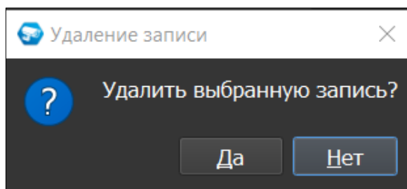
Рисунок 5.32 – Подтверждение удаления
