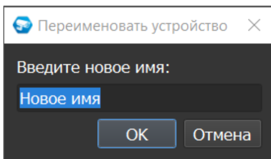
Рисунок 6.57 – Переименовать устройство
