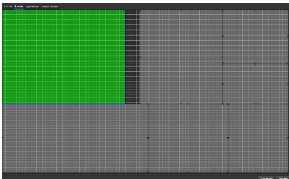
Рисунок 7.48 – Создание раскладки
