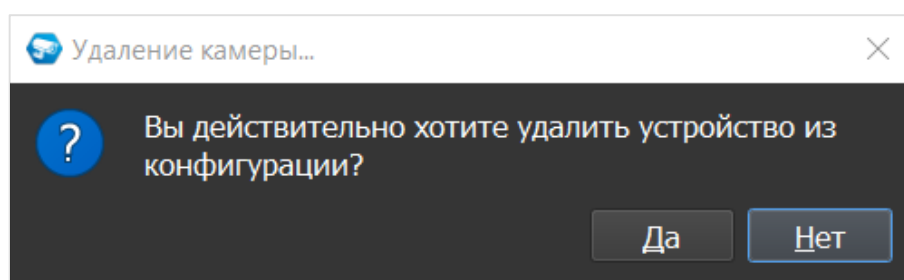
Рисунок 6.55 – Подтверждение
