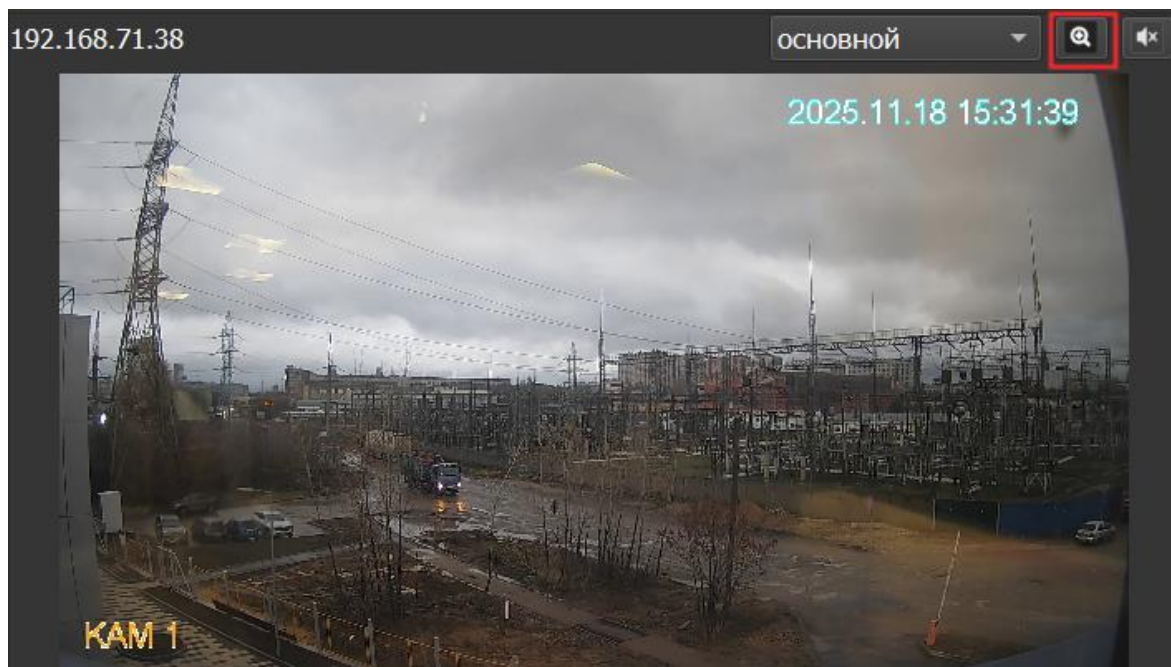
Рисунок 8.19 – Кнопка зума
