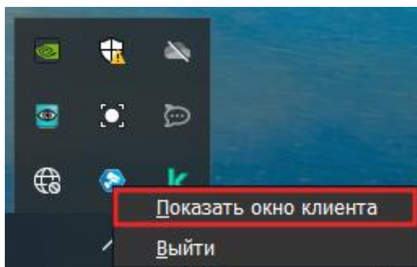
Рисунок 2.25 – Контекстное меню
