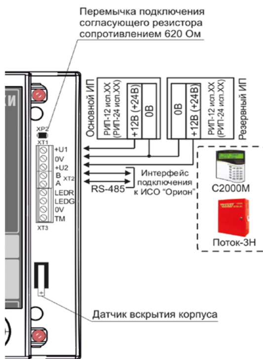
Рисунок 2. Схема внешних соединений блока «Поток-БКИ»
