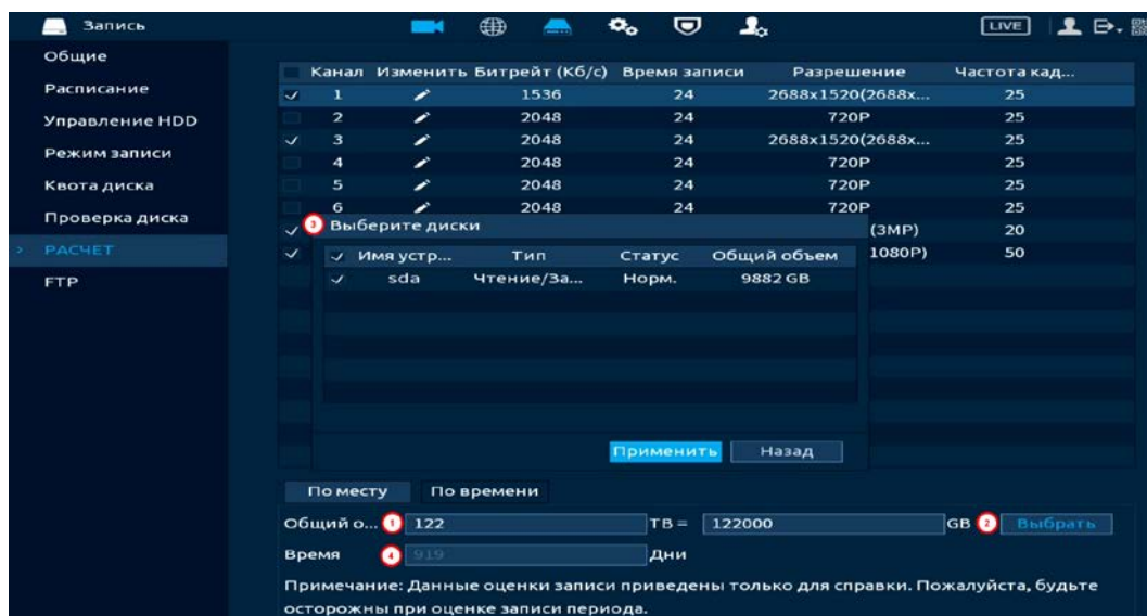
Рисунок 13.21 – Выбор диска для расчёта и результат
