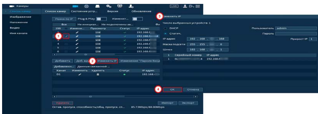
Рисунок 11.20 – Изменения сетевых настроек IP-камер через регистратор
