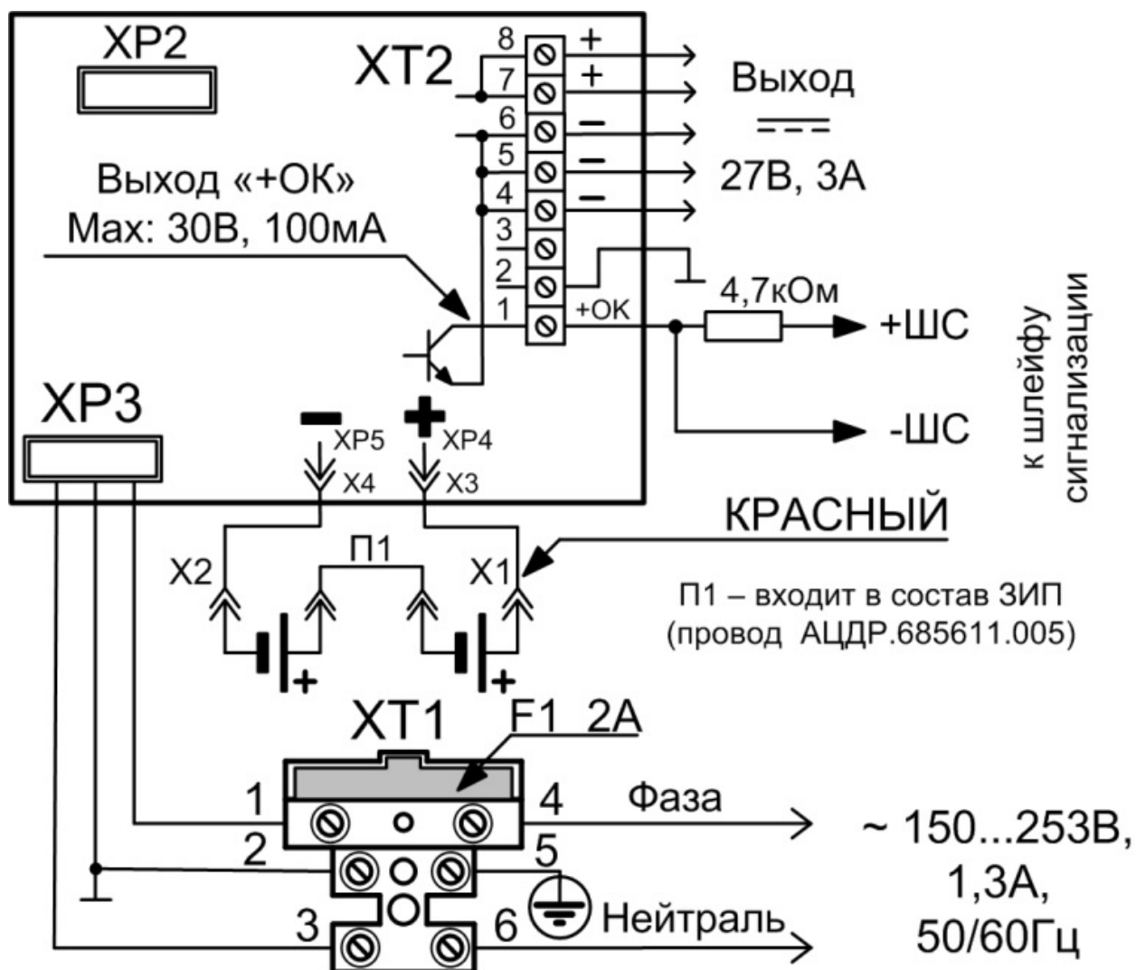
Схема подключения РИП
