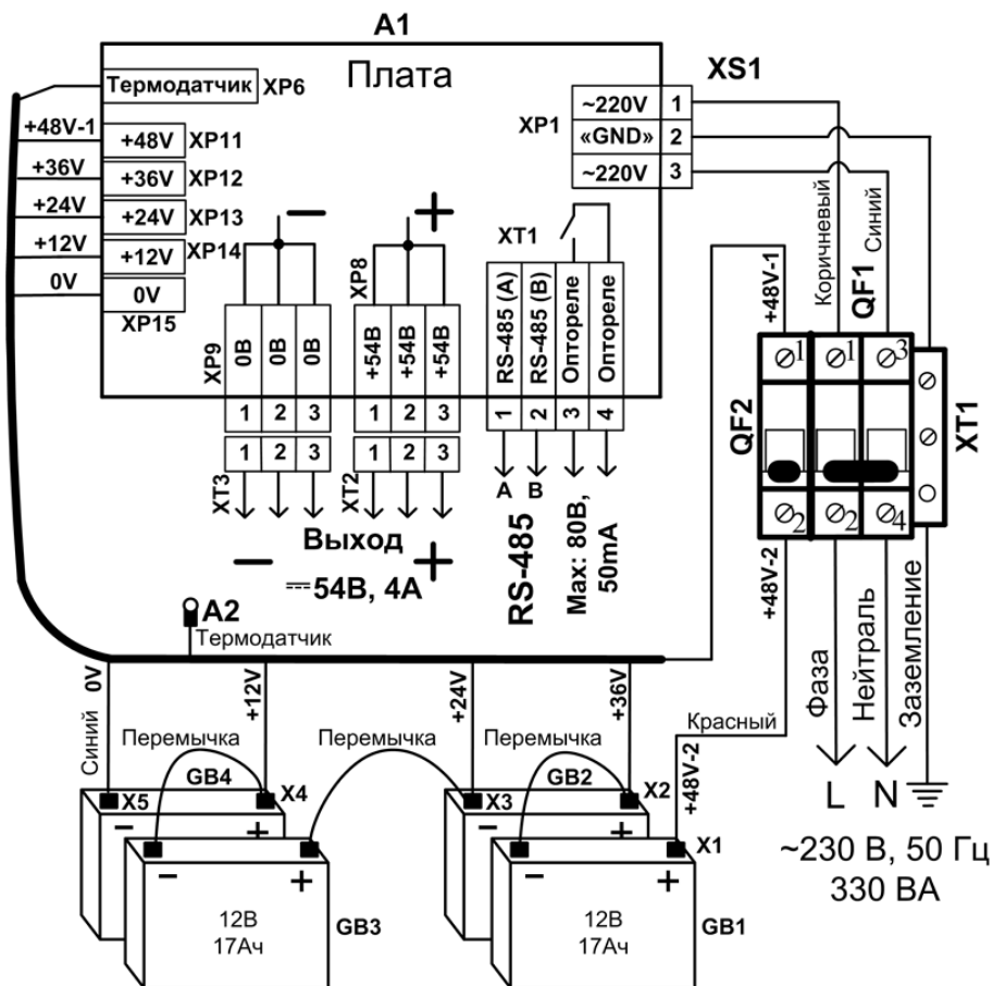
Рисунок 2. Схема соединений.
