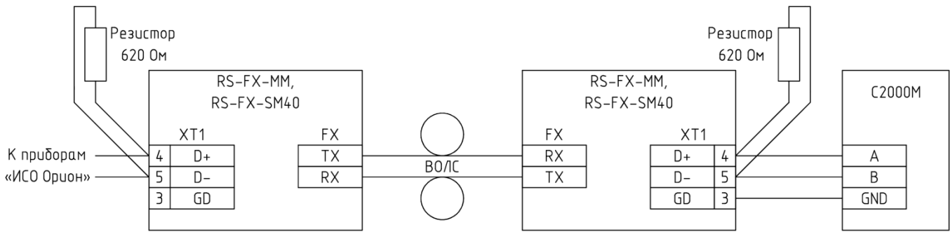
Рисунок 2.2.3 Схема подключения в режиме удлинения RS-485.
