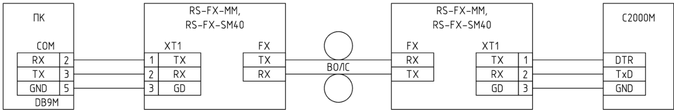
Рисунок 2.2.4 Схема подключения в режиме удлинения RS-232.
