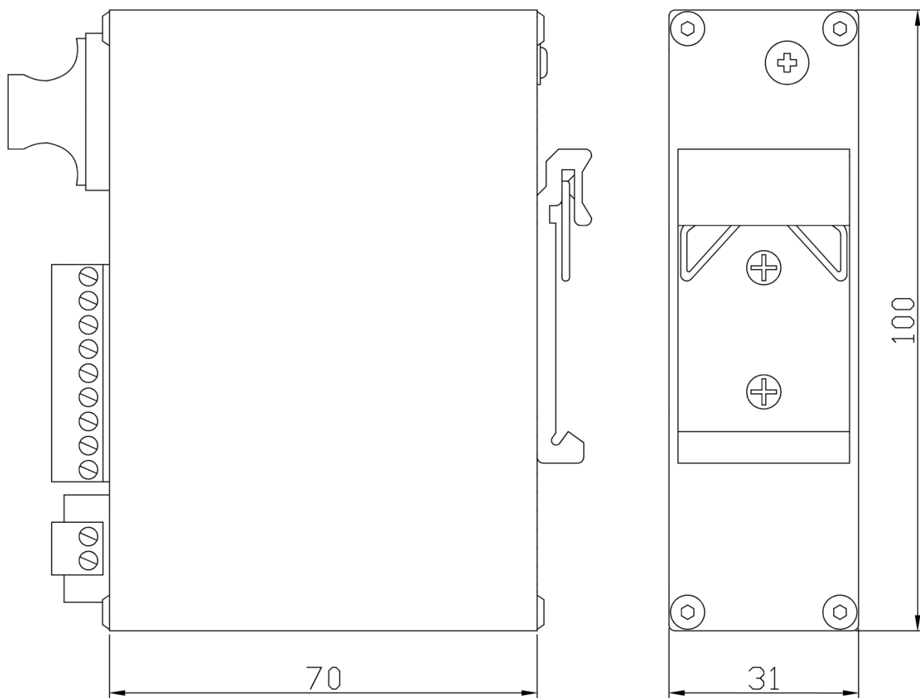
Рисунок 2.2.2 Габаритные размеры преобразователя.
