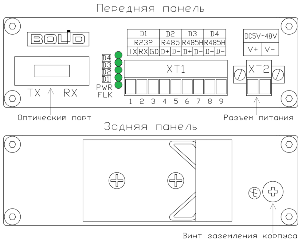
Рисунок 2.2.1 Внешний вид преобразователя.
