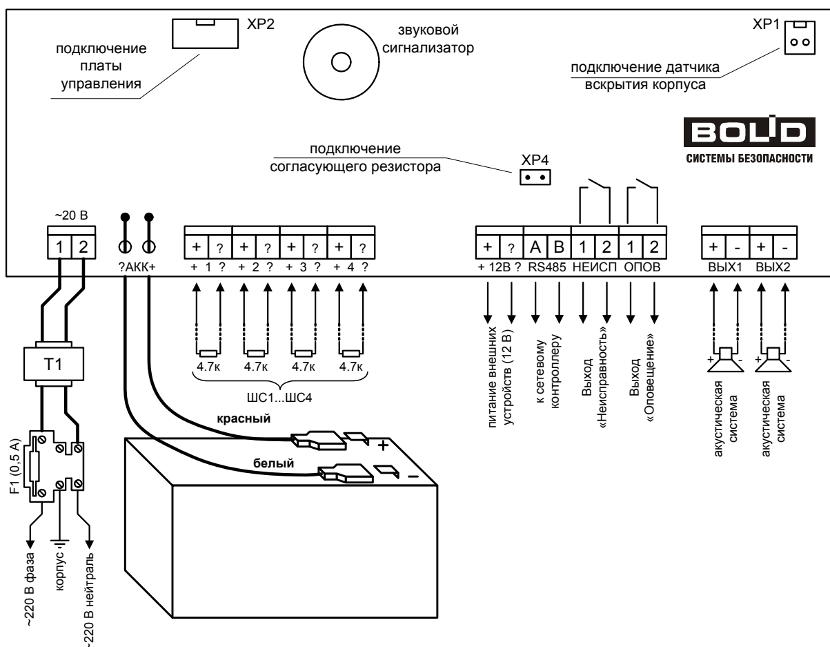
Рисунок 5. Схема подключения прибора
