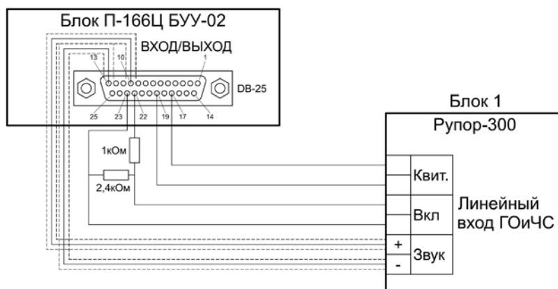
Рисунок 2.5. Схема подключения блока управления П-166Ц БУУ-02.
