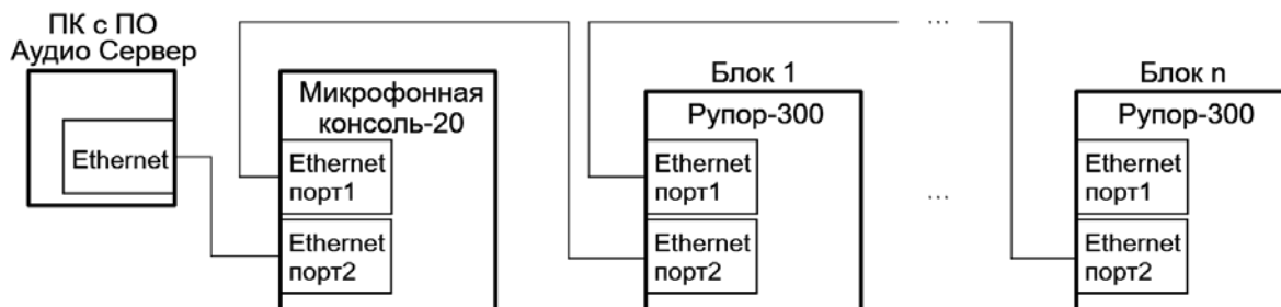
Рисунок 2.7. Схема соединения интерфейсов Ethernet без функции резервирования.
