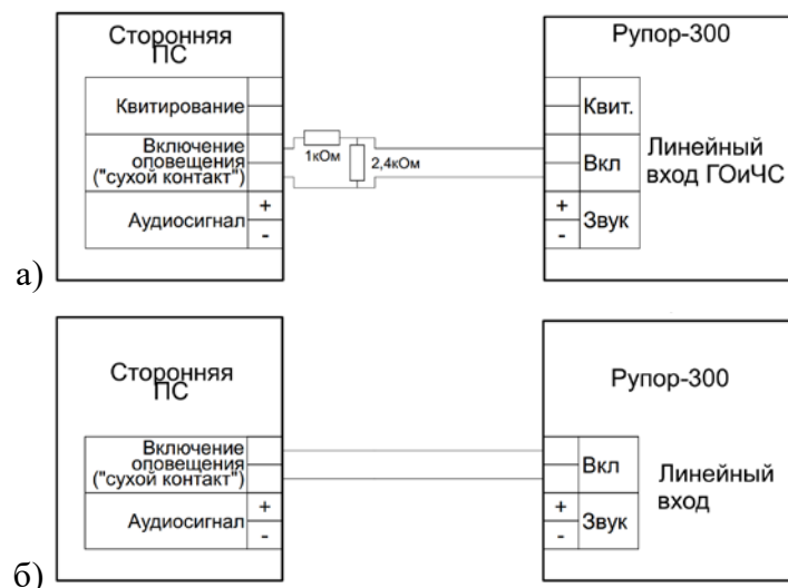
Рисунок 2.8 Подключение сторонней ПС к аналоговому входу для запуска сообщения
