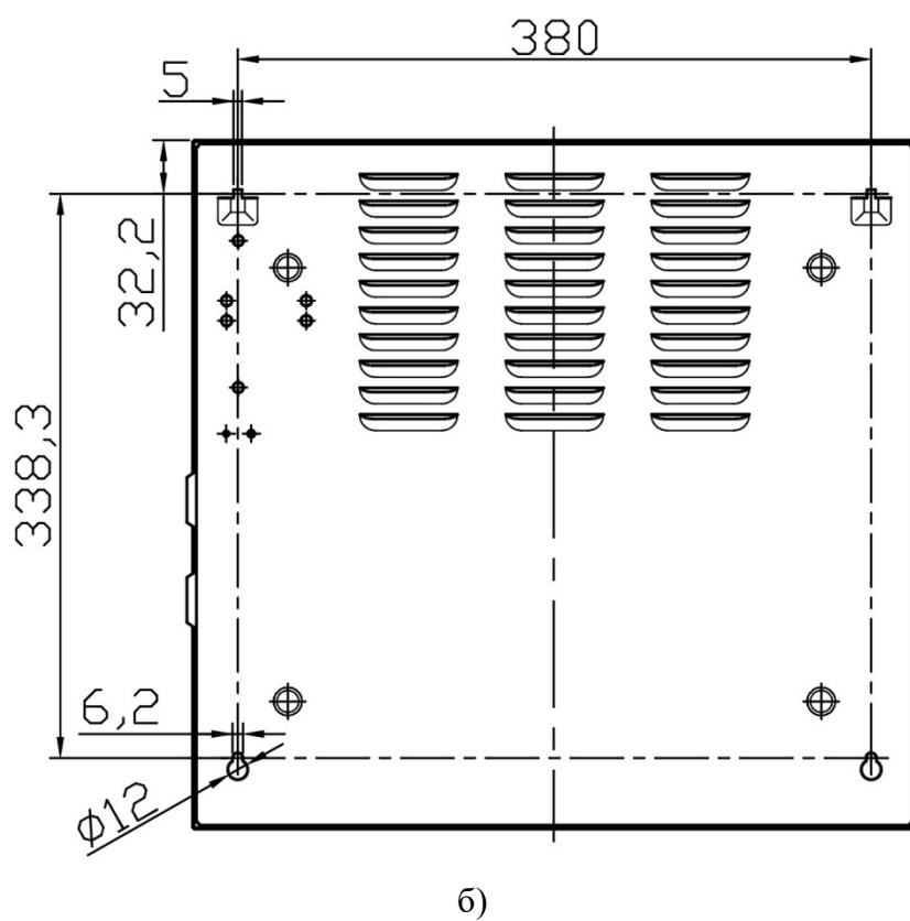
Рисунок 2.2. Габаритные и установочные размеры блока.
