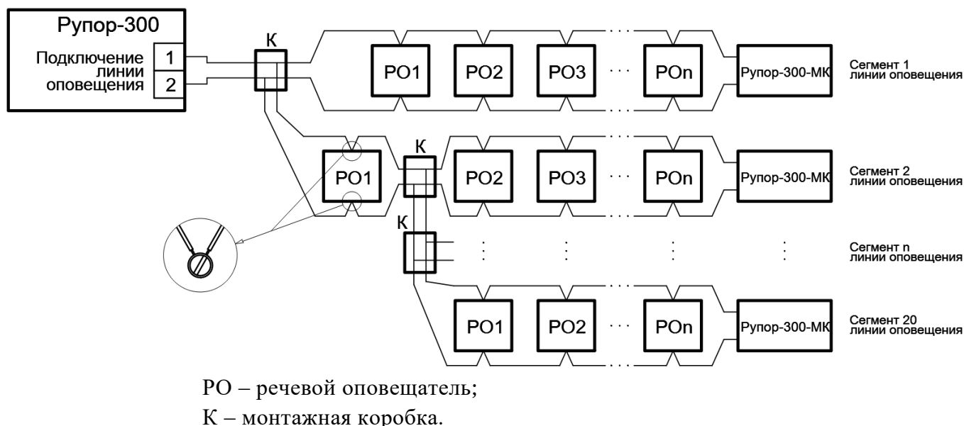
Рисунок 2.9. Подключение громкоговорителей к линиям оповещения
