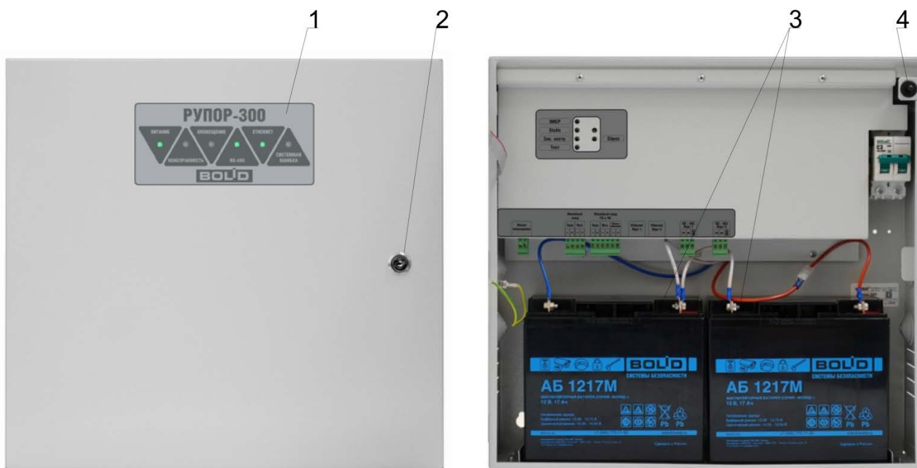
Рисунок 2.1. Внешний вид блока.
