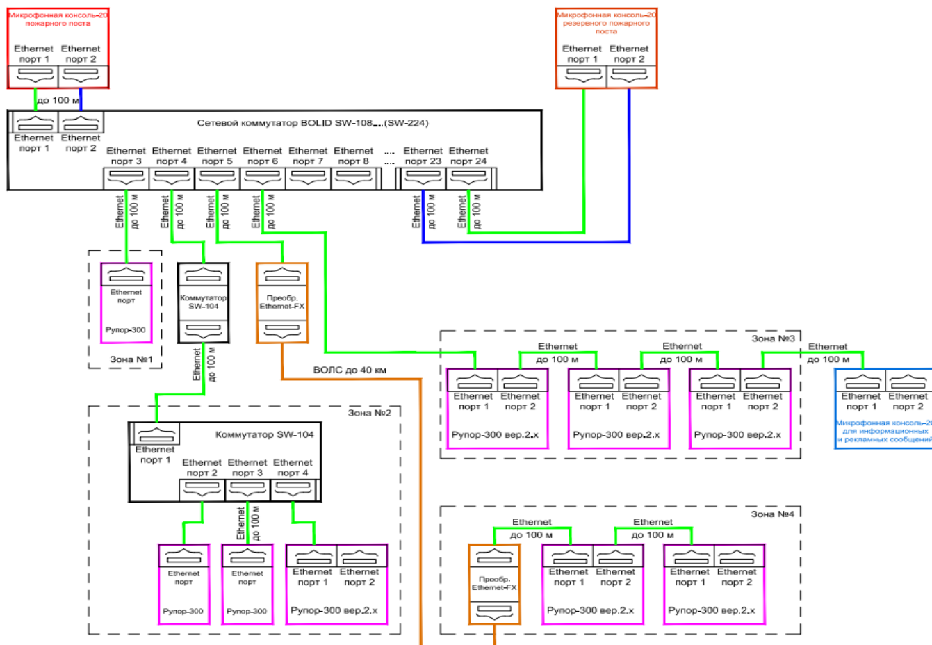
Рисунок 2.6. Схема организации сети для совместной работы устройств.
