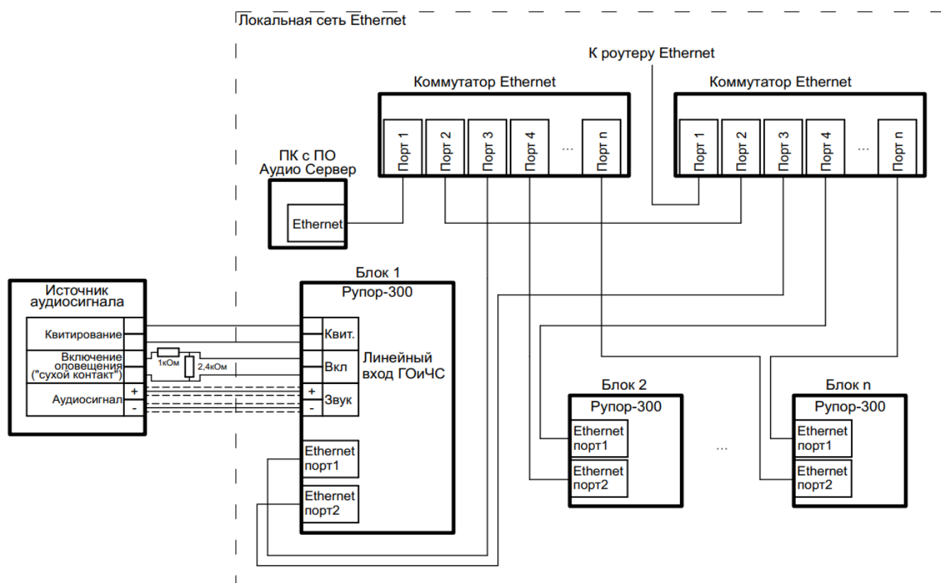
Рисунок 2.4. Схема подключения источника сигнала ГОиЧС и резервирования Ethernet.
