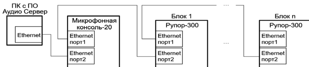
Рисунок 2.7. Схема соединения интерфейсов Ethernet без функции резервирования.
