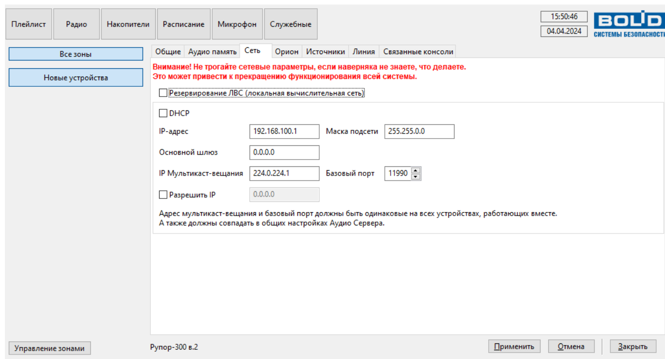
Рисунок 2.2.15. Настройки сетевых подключений блока
