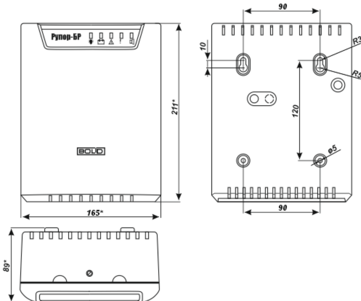
Рис. 3 Габаритные и установочные размеры
