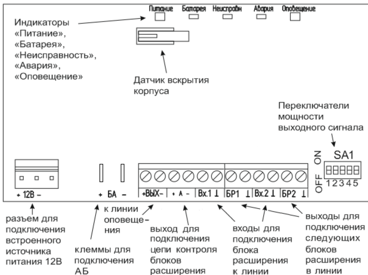
Рис. 1 Плата «Рупора-БР 2RS485»
