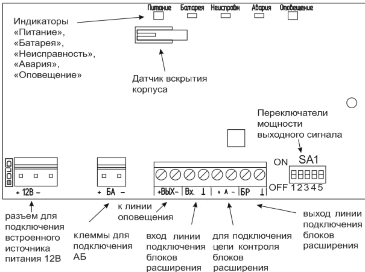
Рис. 2 Плата «Рупора-БР»
