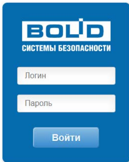
Рисунок 6-1 Окно аутентификации
