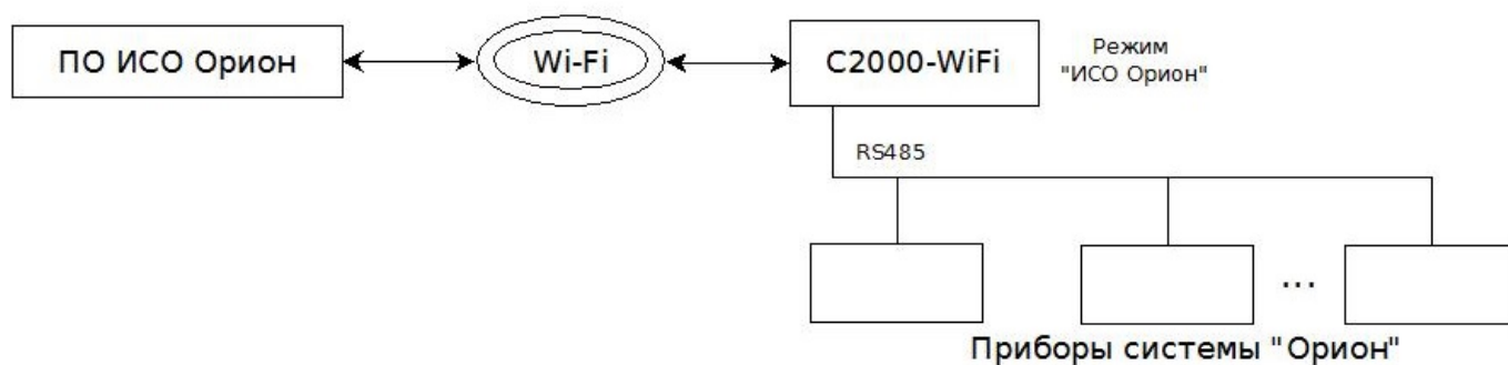
Рисунок 2.6. Подключение «C2000-WiFi» по протоколу «Орион».
