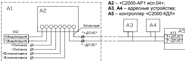
Рисунок 1 Схема соединений
