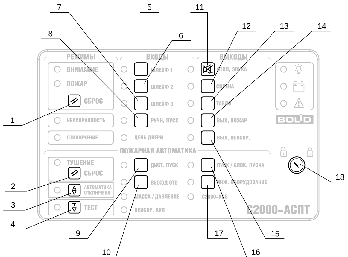
Рисунок 2. Расположение кнопок
